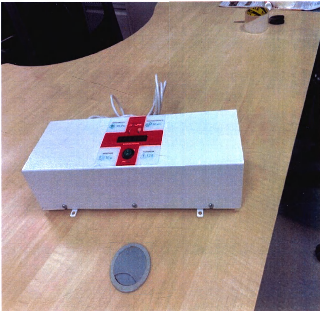
Рис.1.3. Облучатель - рециркулятор воздуха ультрафиолетовый бактерицидный U-1A по ТУ 32.50.50-019-47272295-2021
