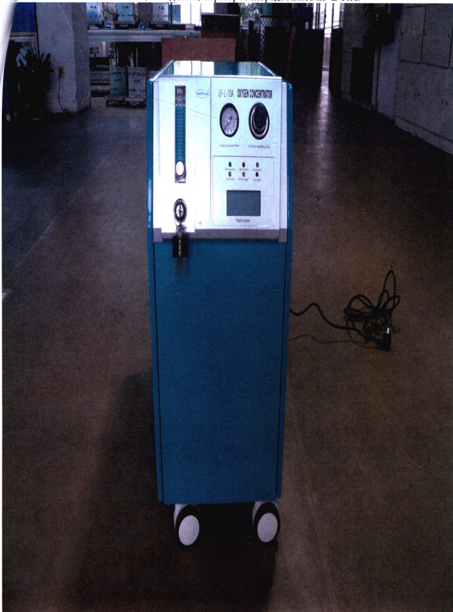
Общий вид Концентратор кислорода Armed LF-L-10A.
