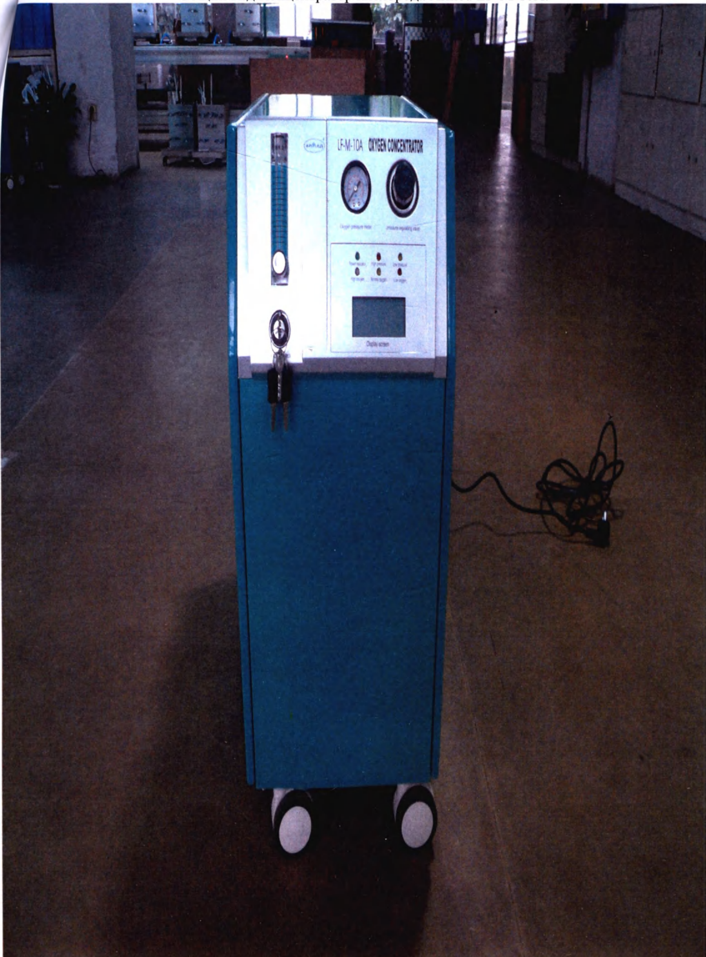
Общий вид Концентратор кислорода Armed LF-M-10A.
