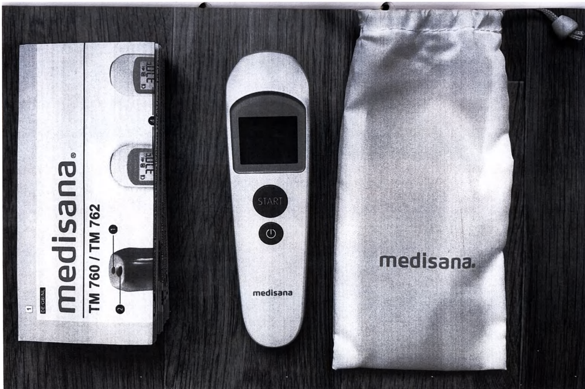
Общий вид Термометра медицинского инфракрасного Medisana TM 760
