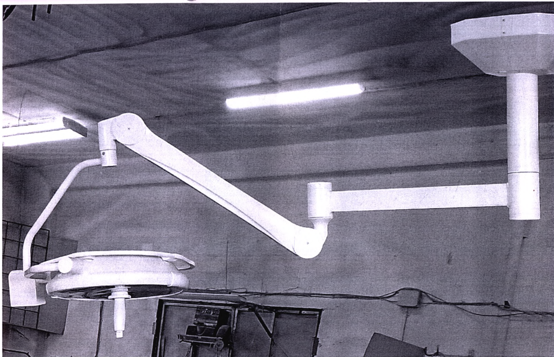
Рисунок 3 – Светильник медицинский операционный (хирургический) «Люмэс-ОС-500-П-800/800»
