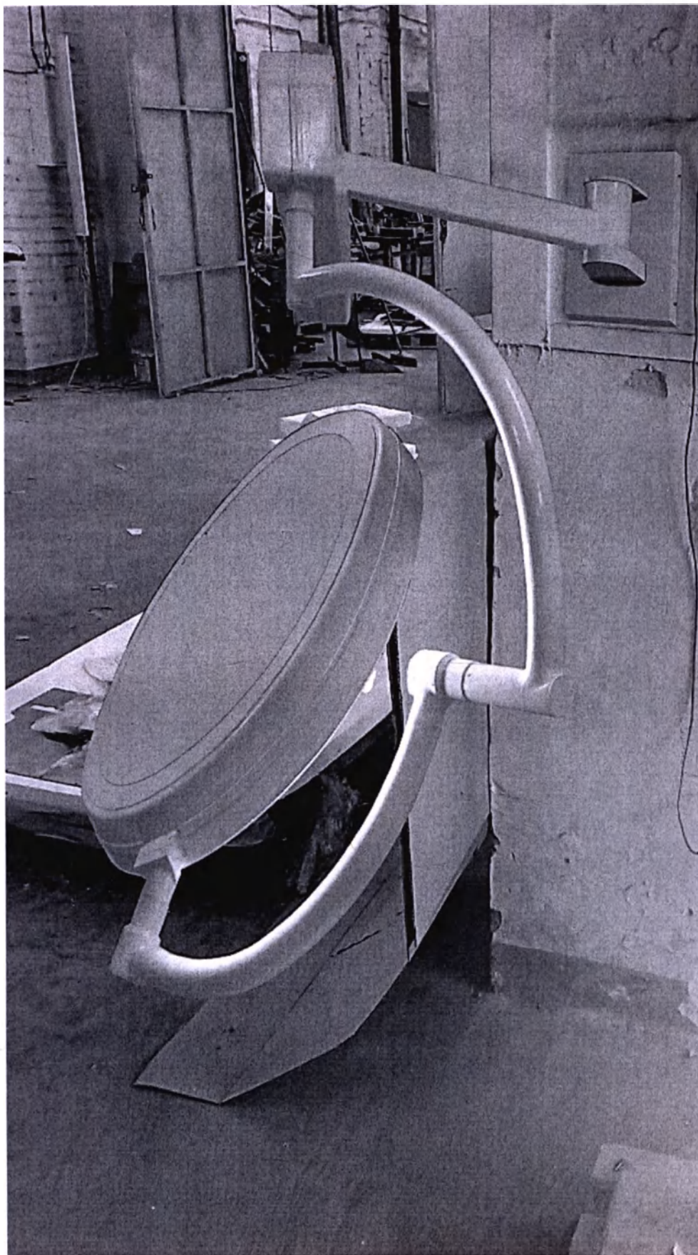
Рисунок 13 – Светильник медицинский операционный (хирургический) «Люмэс-ОС-800-С-800/800»
