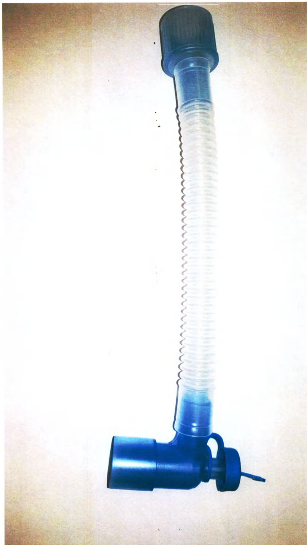
24. Соединитель угловой гофрированный 170 мм, 22F-15F/22М, с портом 9,5 мм
