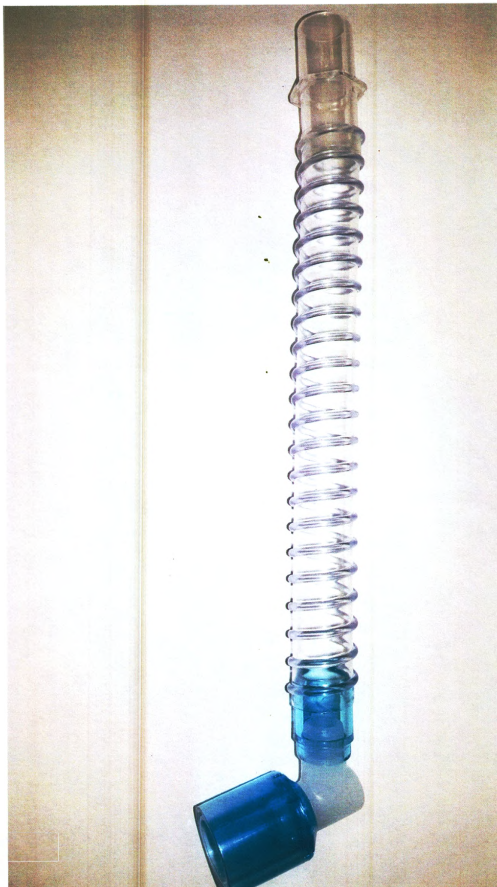
91. Соединитель угловой гладкоствольный 170 мм, 15М-15F/22М, шарнирный
