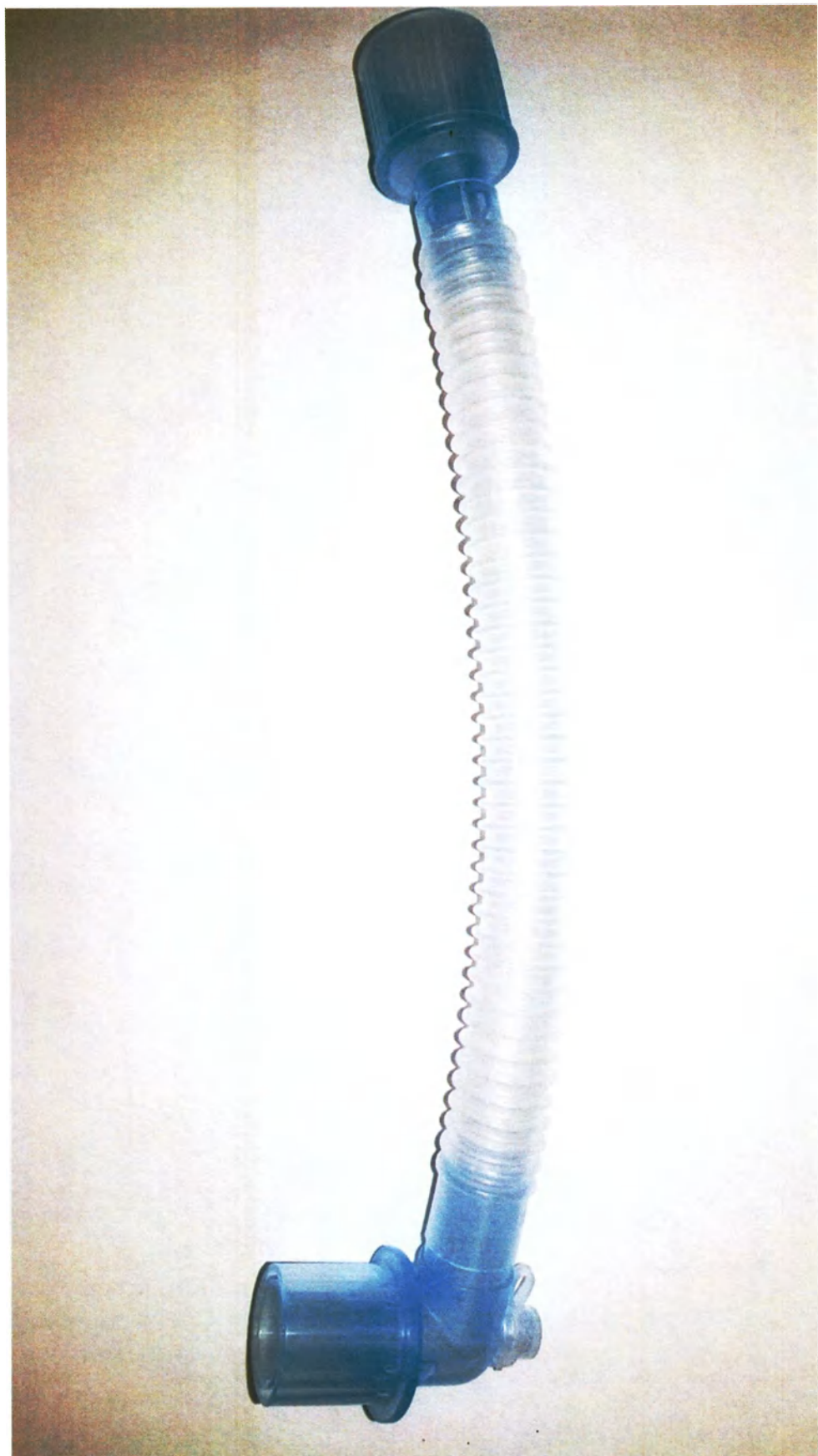
30. Соединитель угловой гофрированный 230 мм, 22F-15F/22М, с портом Луер-Лок
