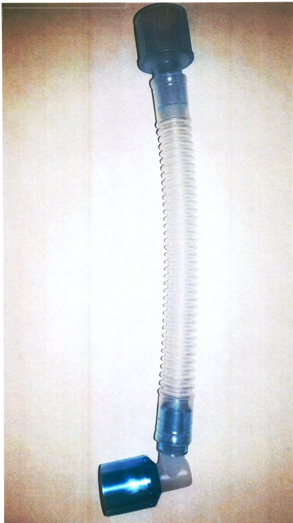
36. Соединитель угловой гофрированный 170 мм, 22F-15F/22М, шарнирный
