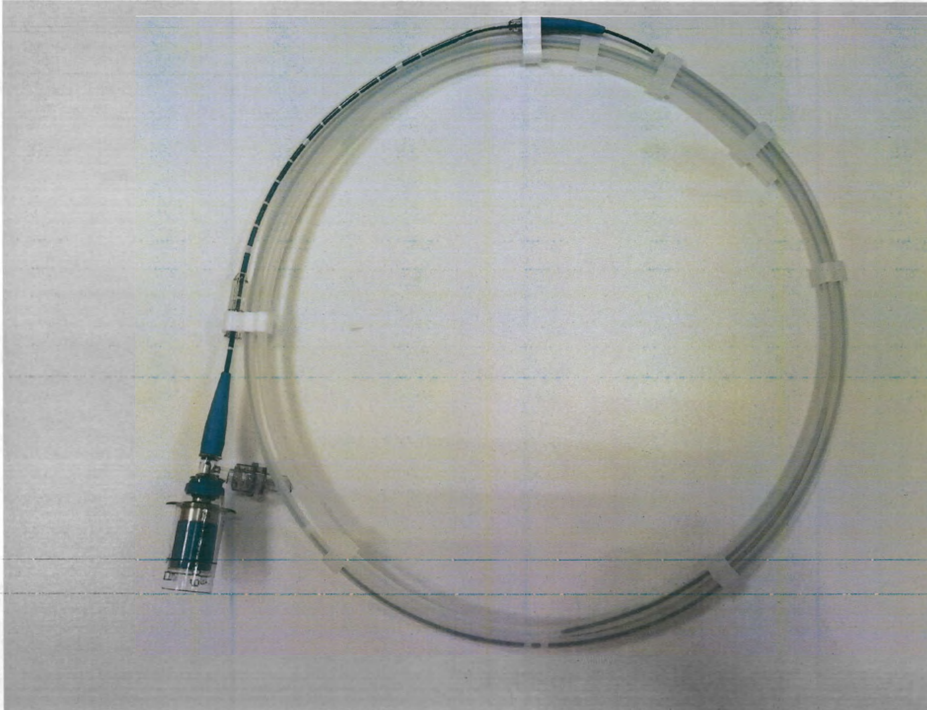
Общий вид катетера для васкулярной визуализации OptiCross 18 30 МГц в защитной трубке с зажимами
