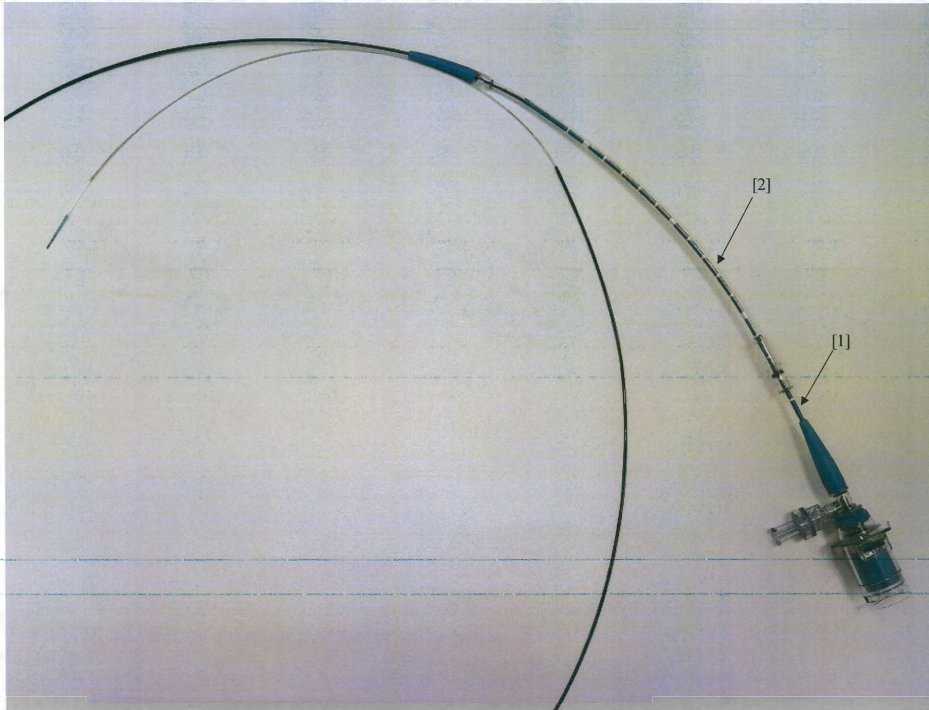
Внутренняя телескопическая трубка [1], наружная телескопическая трубка [2]
