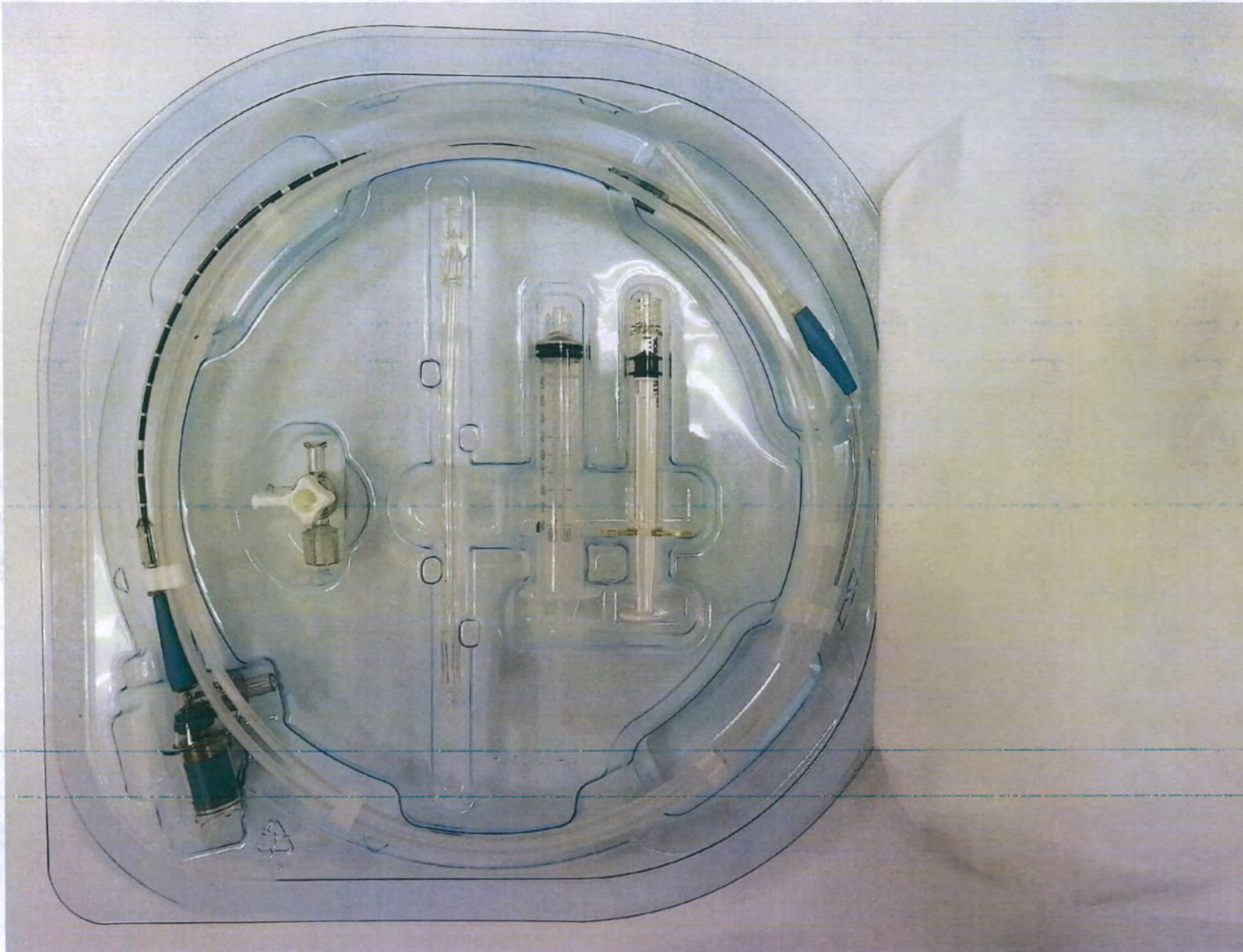
Общий вид катетера для васкулярной визуализации OptiCross 35 15 МГц в составе в индивидуальной упаковке (лотке)
