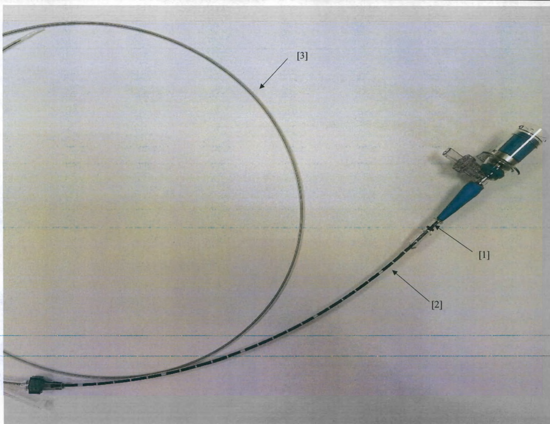
Внутренняя телескопическая трубка [1], наружная телескопическая трубка [2], трубка с просветом для проводника [3]
