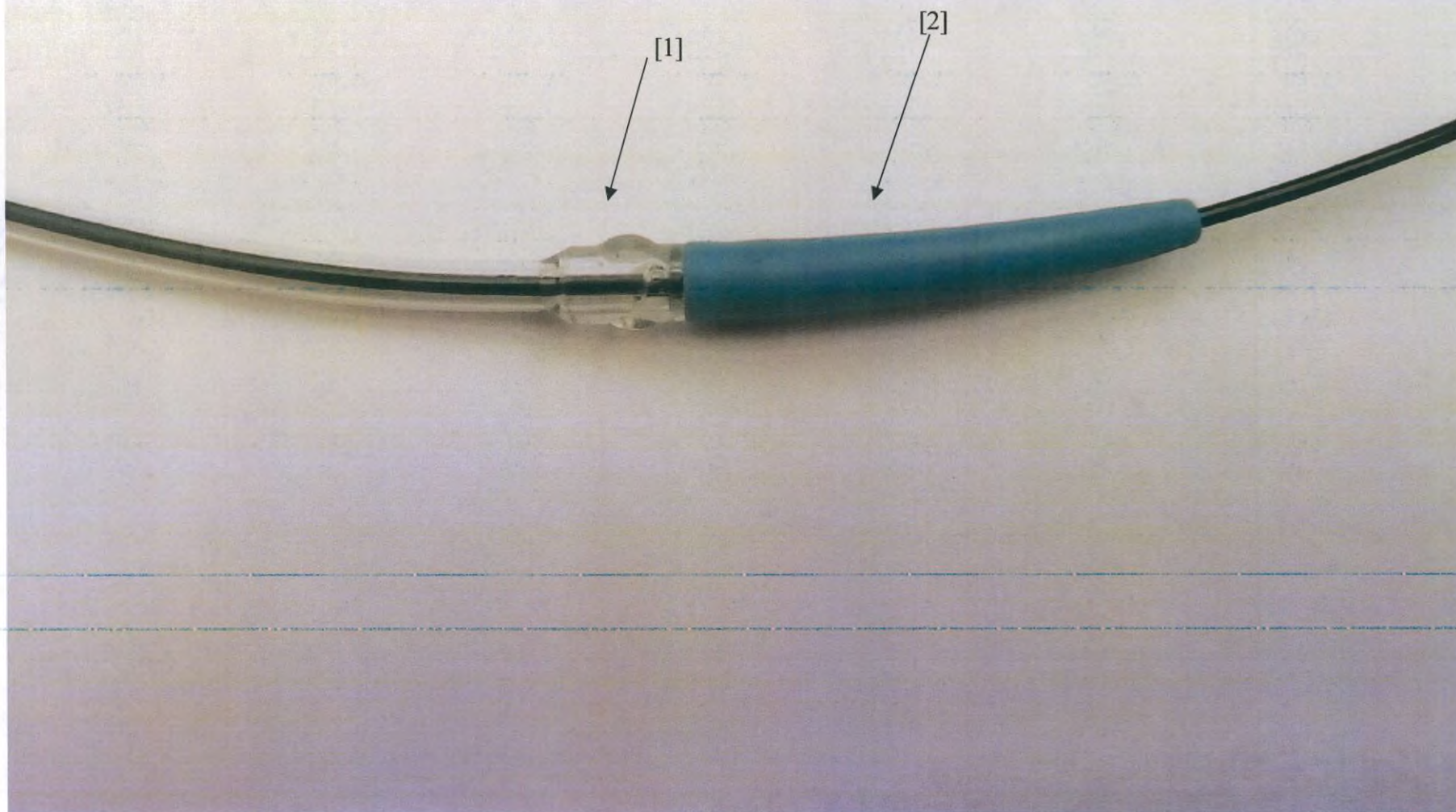
Держатель разгрузочной муфты [1], дистальная разгрузочная муфта [2]
