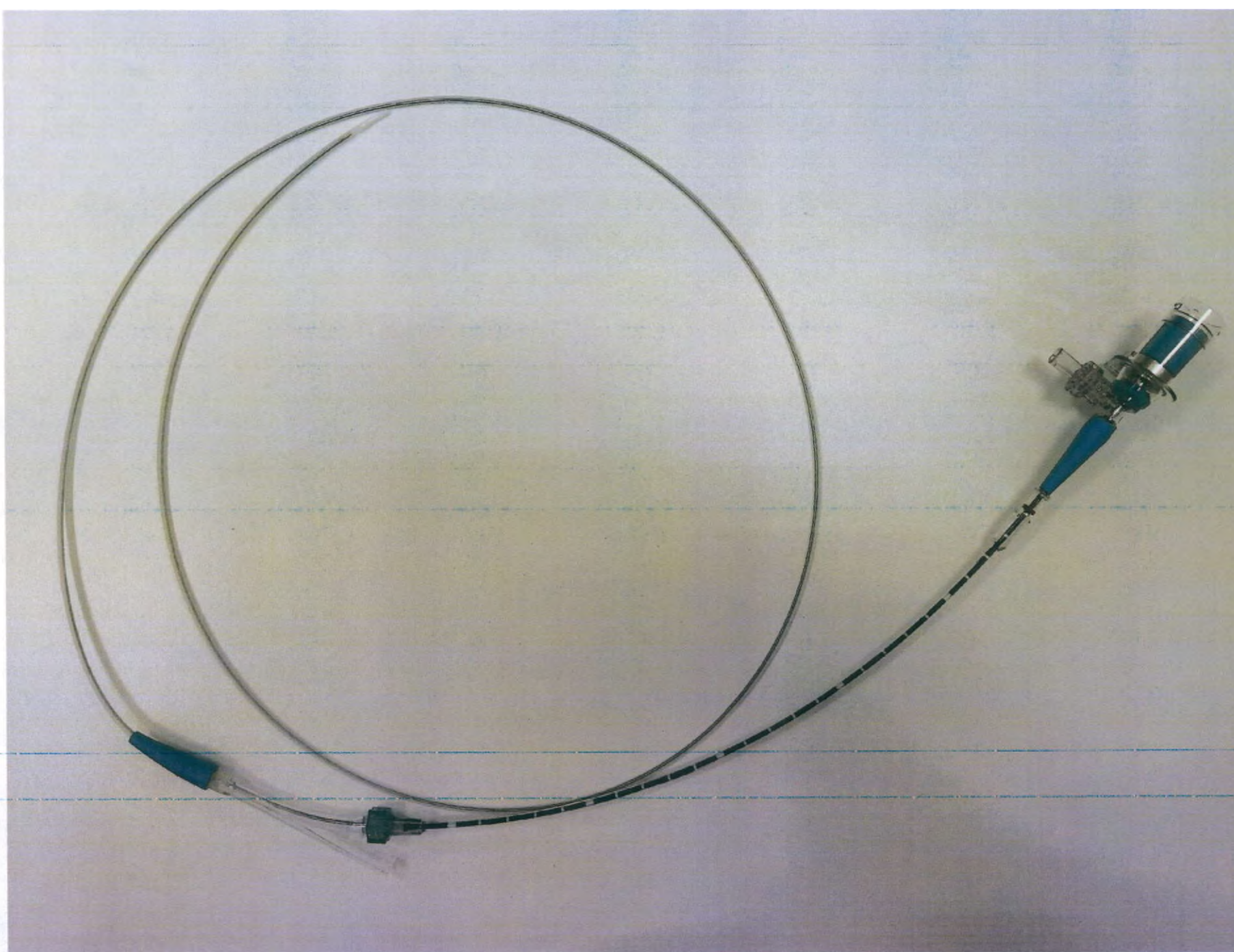
Катетер для васкулярной визуализации OptiCross 35 15 МГц
