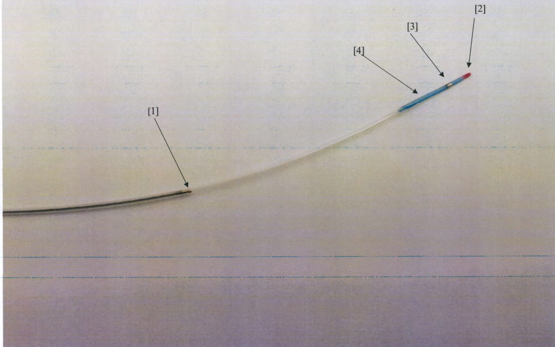
Пьезоэлектрический датчик [1], дистальный кончик [2], рентгеноконтрастная метка [3] и трубка с просветом для проводника [4]
