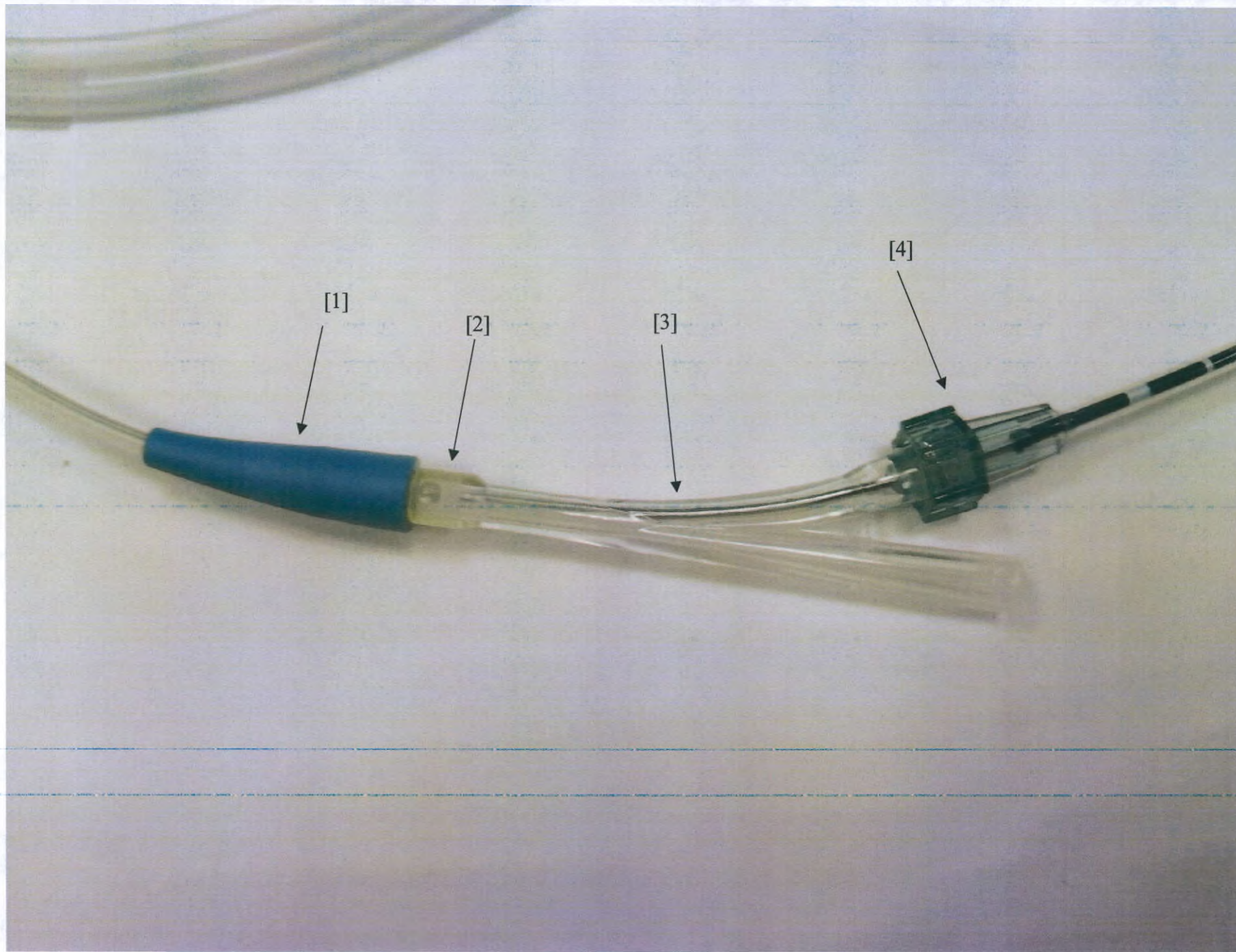
Дистальная разгрузочная муфта [1], держатель разгрузочной муфты [2], Y-образный коннектор [3] и разъем Люэра [4]
