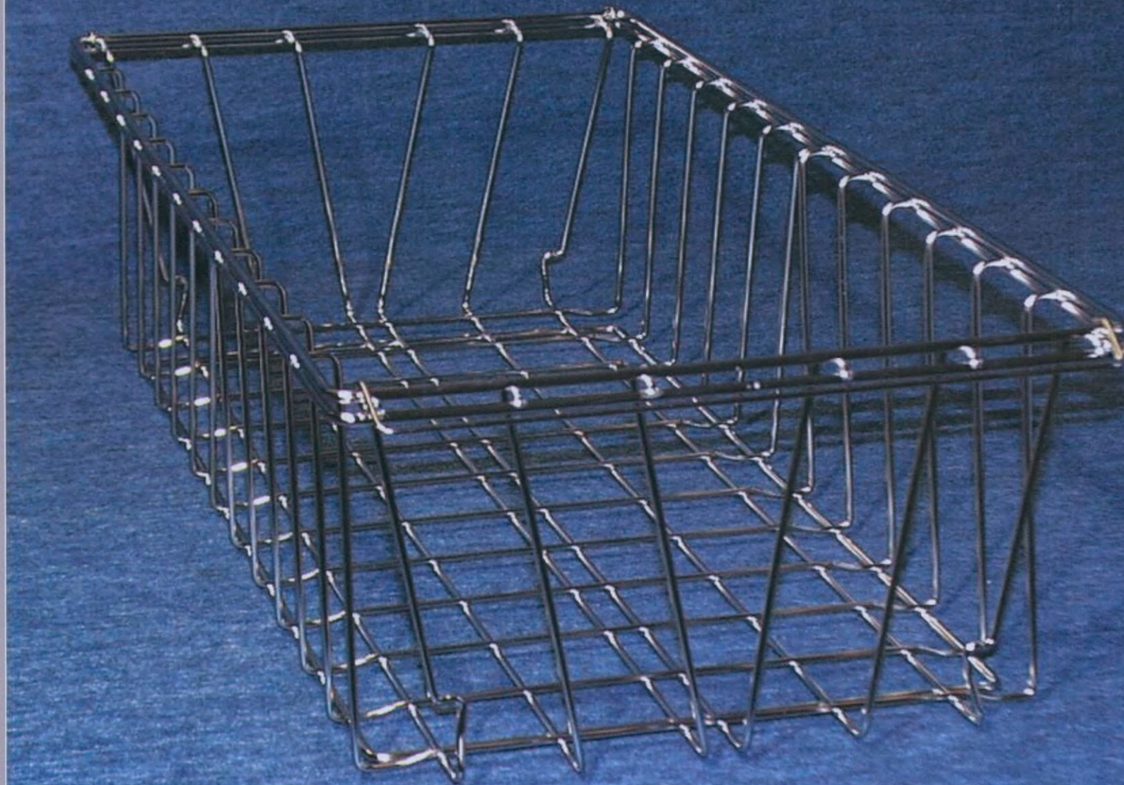
Корзина проволочная ( размеры: 300х600х300 мм)
