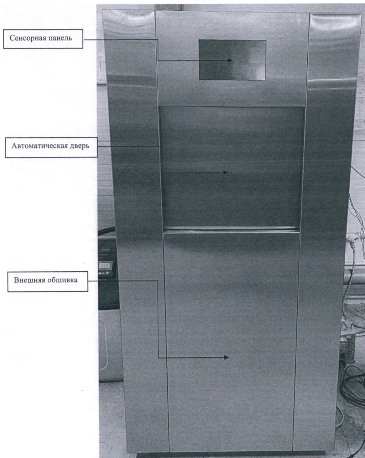
Рисунок 1а – Общий вид стерилизатора со стороны зоны выгрузки. (Для двухдверного стерилизатора)
