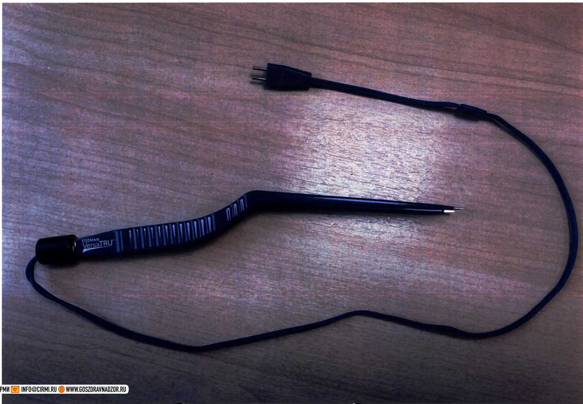
Биполярный пинцет CODMAN VersaTru®, длина 230 мм, наконечник 1.0 мм
