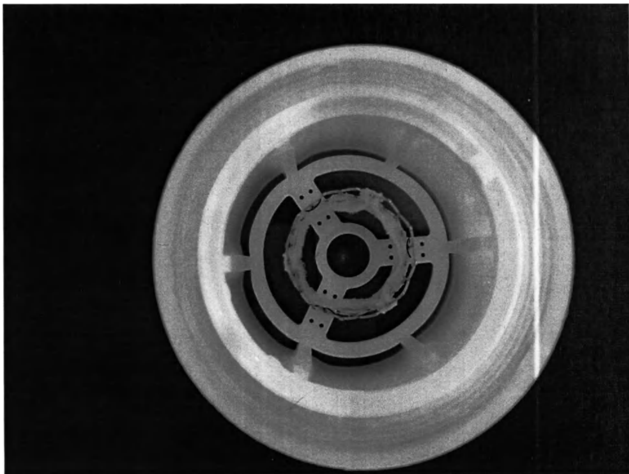
Фото 4. Каркас (кейдж), содержащий клапан «Клапан аортальный транскатетерный Myval™ (Myval™ Transcatheter Heart Valve)», помещают в ПП банку (контейнер). Каркас помещен в банку ПП (контейнер)
