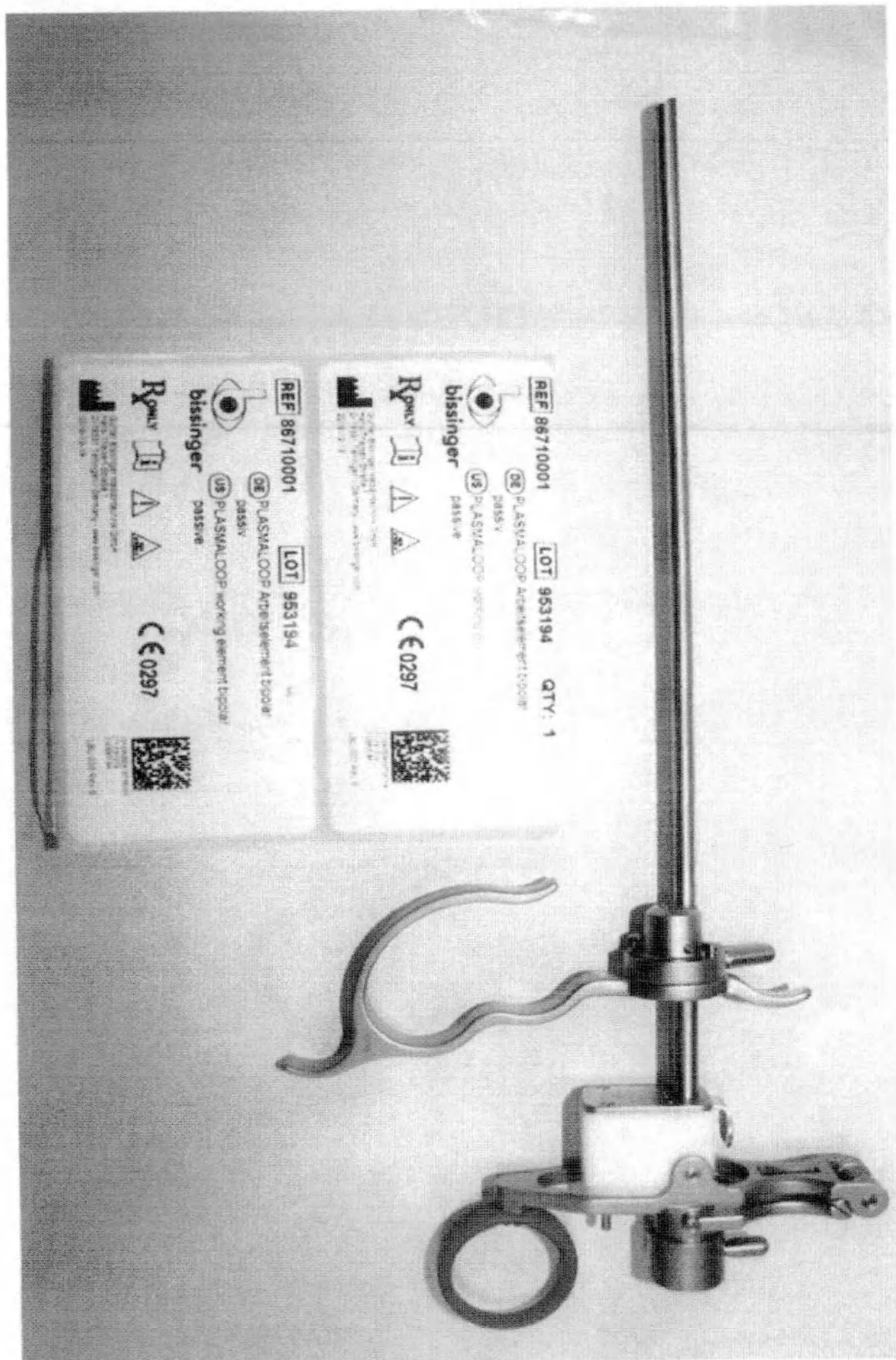
Рабочий элемент, пассивный, биполярный 86710001
