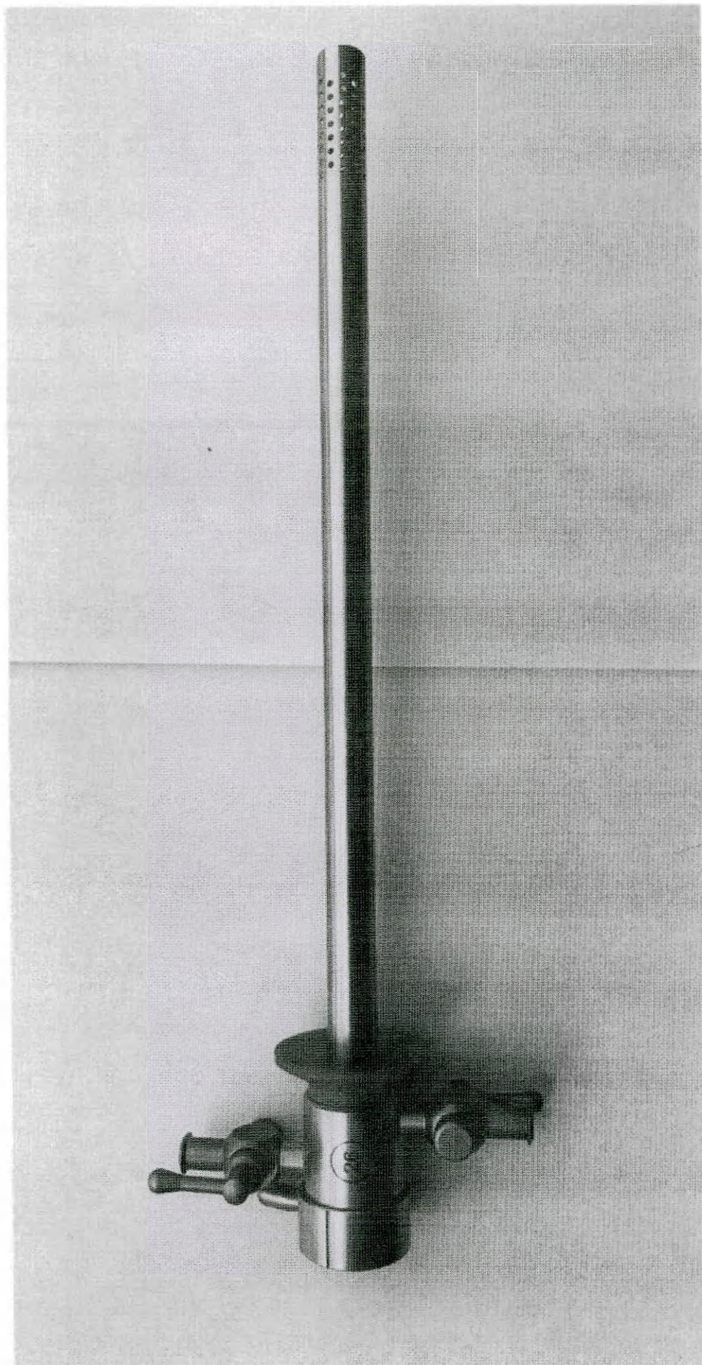
Внешняя трубка тубуса с двумя соединительными трубками и кранами для подачи и отвода жидкости, поворотная, 26 Fr, 86710038
