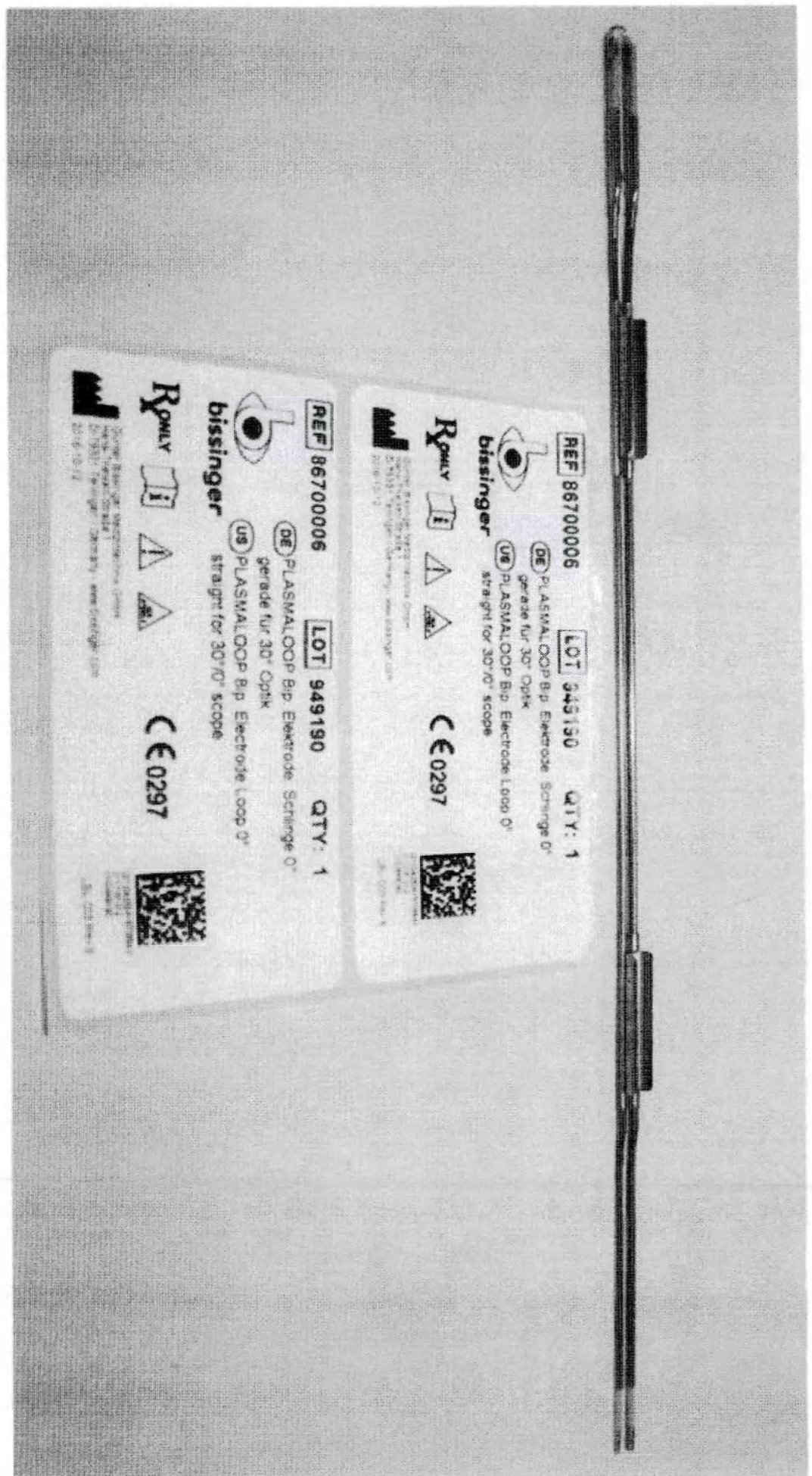
Электрод в форме петли 0°, 86700006.
