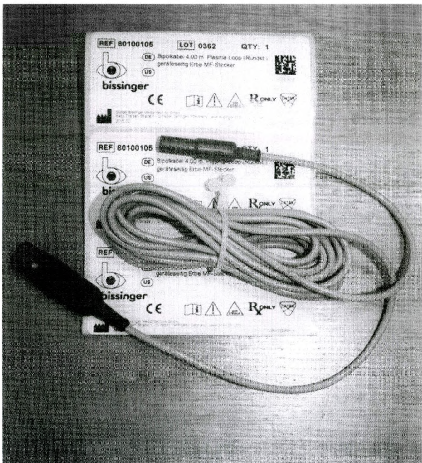
Штекер совместимый с генератором Erbe MF (только для PLASMALOOP) длиной 4 м, 80100105.
