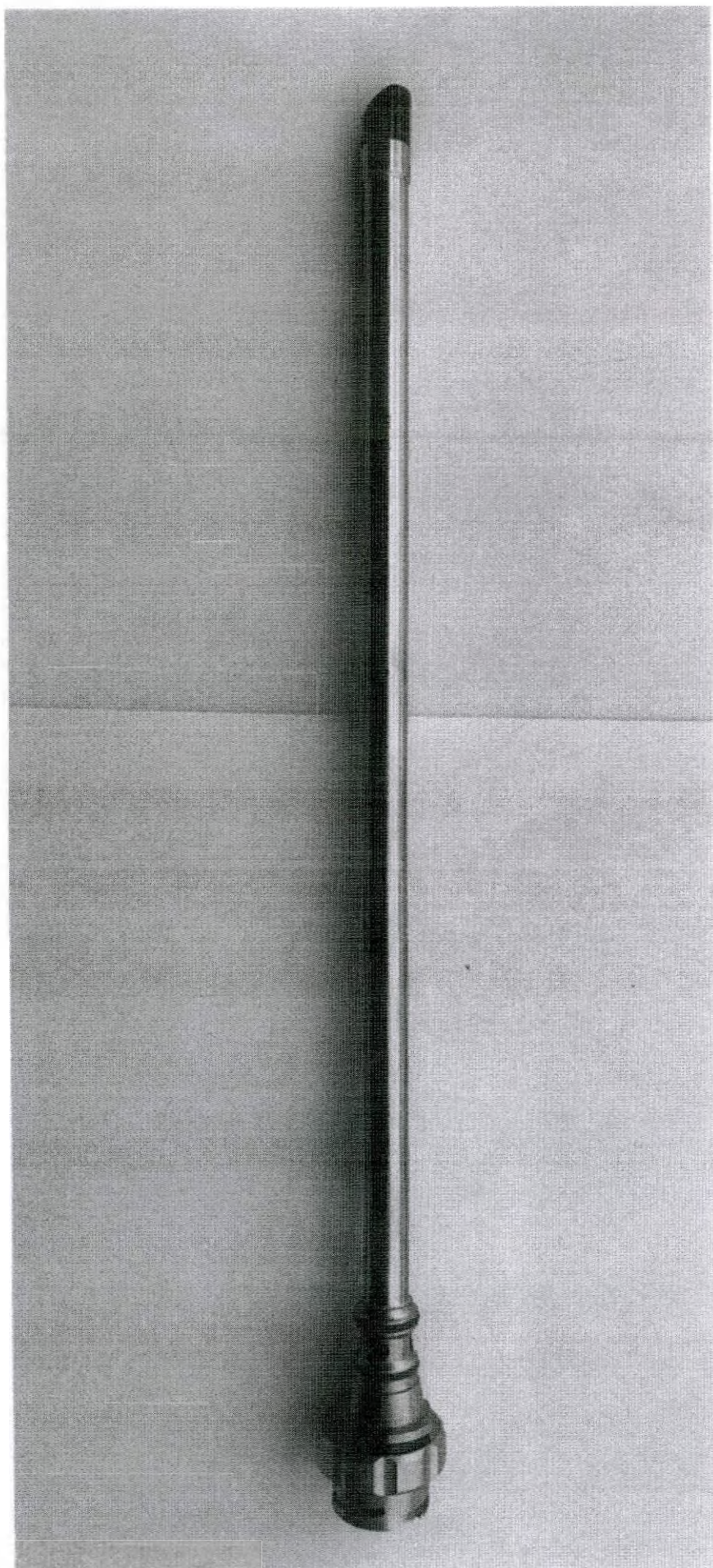
Внутренняя трубка тубуса с керамическим наконечником, поворотная, 24 Fr, 86710039.
