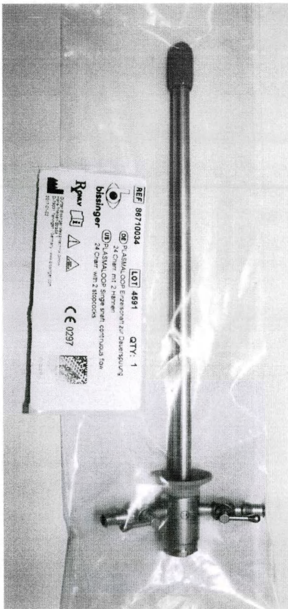
Тубус с двумя соединительными трубками и кранами для подачи и отвода жидкости неповоротный, 24 Fr, 86710034
