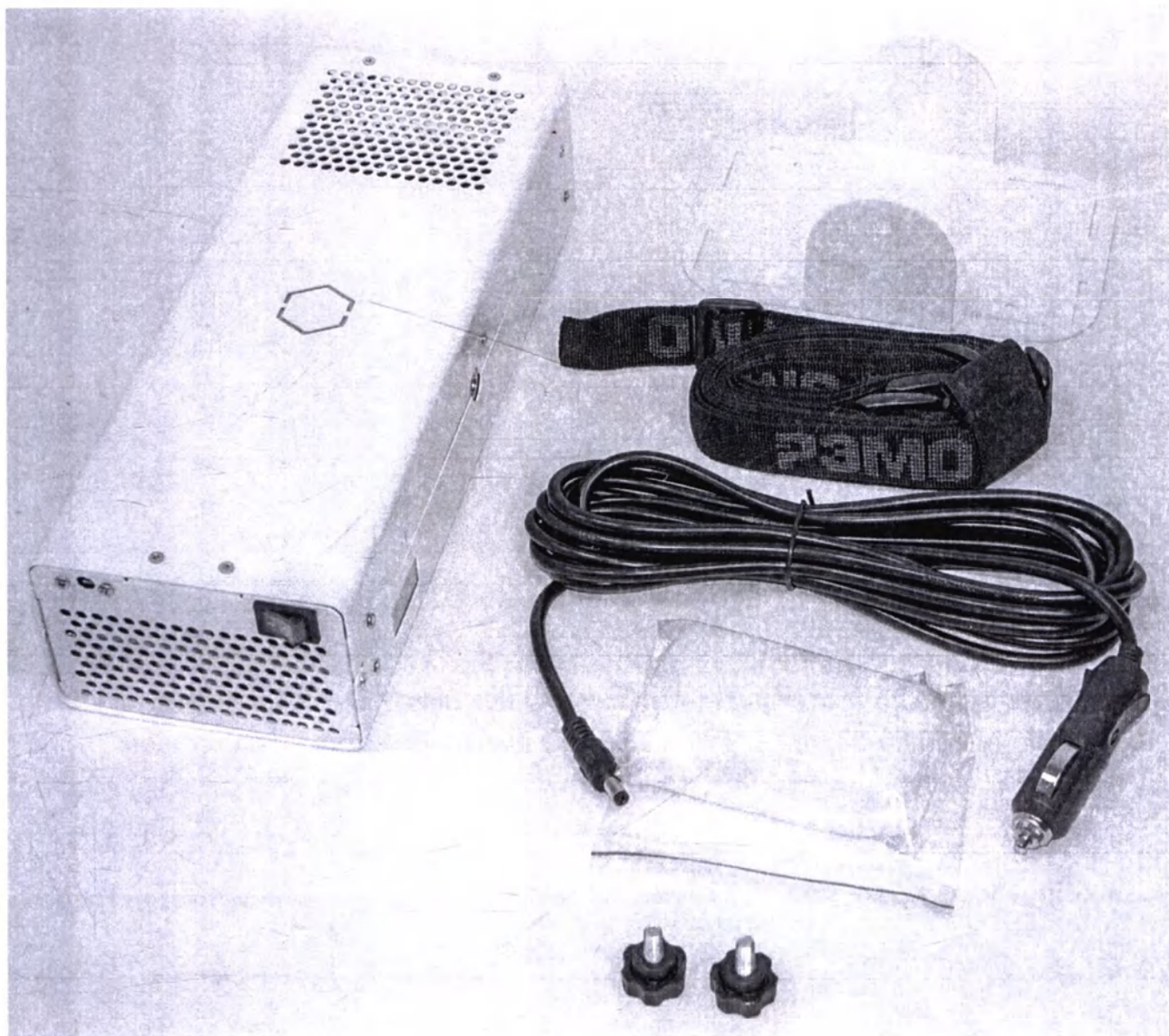
Рисунок 1.1 – Облучатель-рециркулятор бактерицидный медицинский автомобильный ОВУ-21 по ТУ 32.50.50-004-13760586-2020
