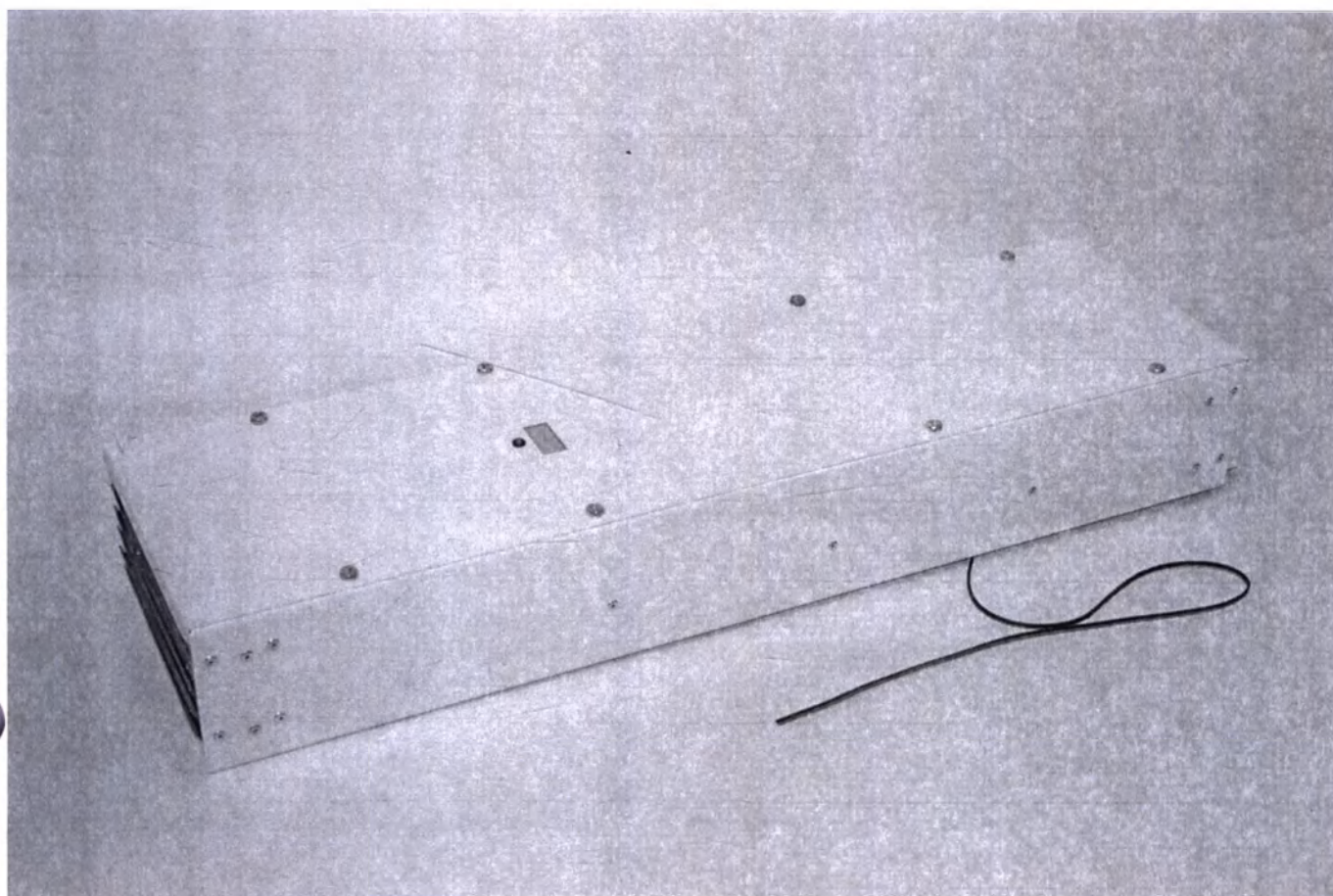
Рисунок 3.1 – Облучатель-рециркулятор бактерицидный медицинский автомобильный ОВУ-24 по ТУ 32.50.50-004-13760586-2020
