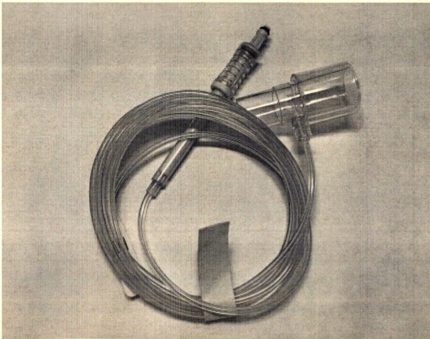
Линия образца одноразовая для опции капнографии
