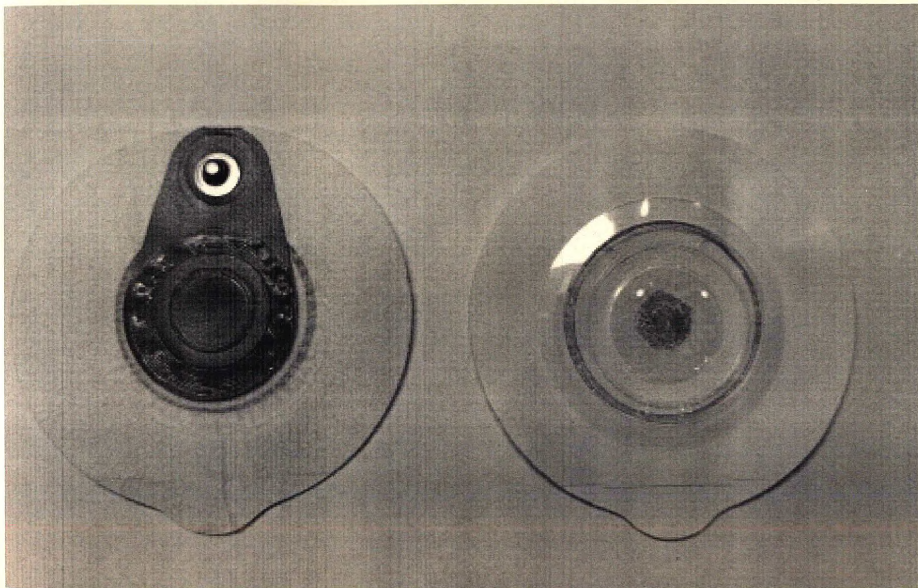
Комплект ЭКГ электродов, Ambu BlueSensor
