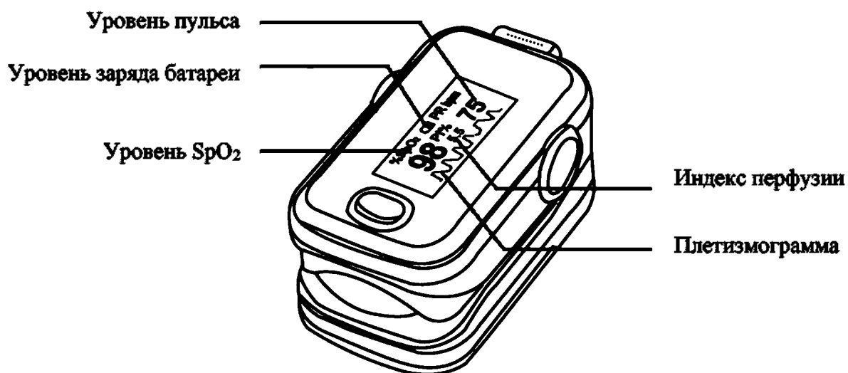
Рис. 3. Дисплей прибора
