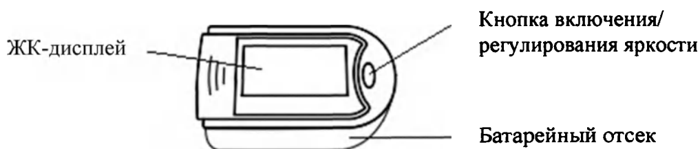
Рис. 2. Элементы прибора
