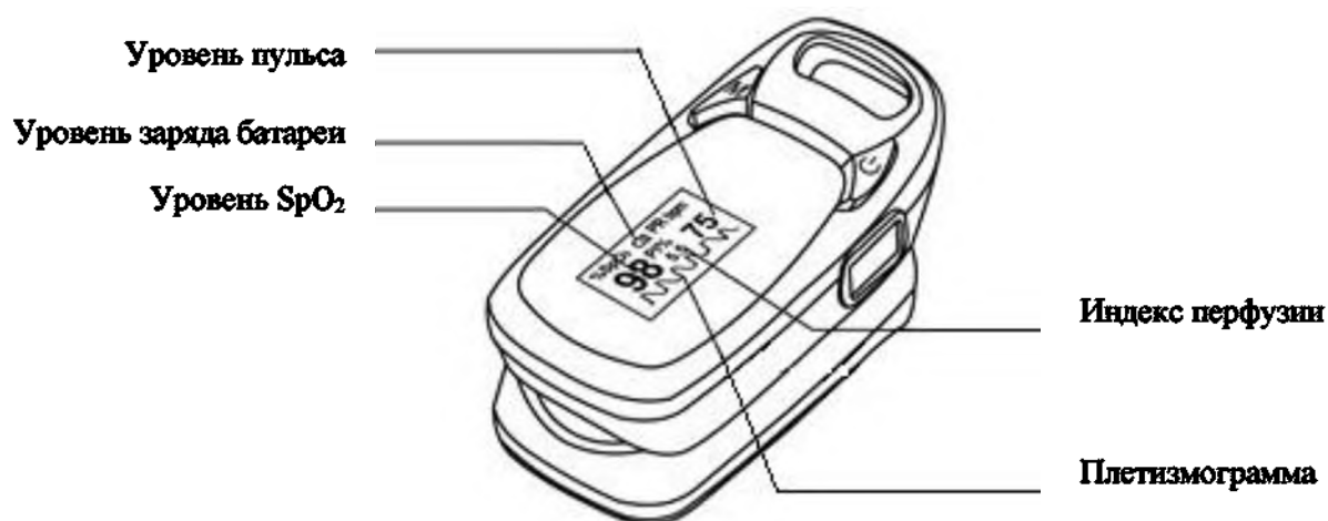
Рис. 3. Дисплей прибора
