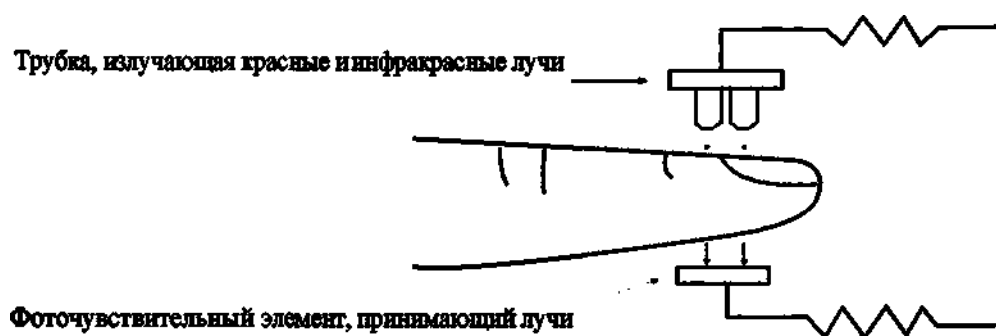
Рис. 1. Принцип работы
