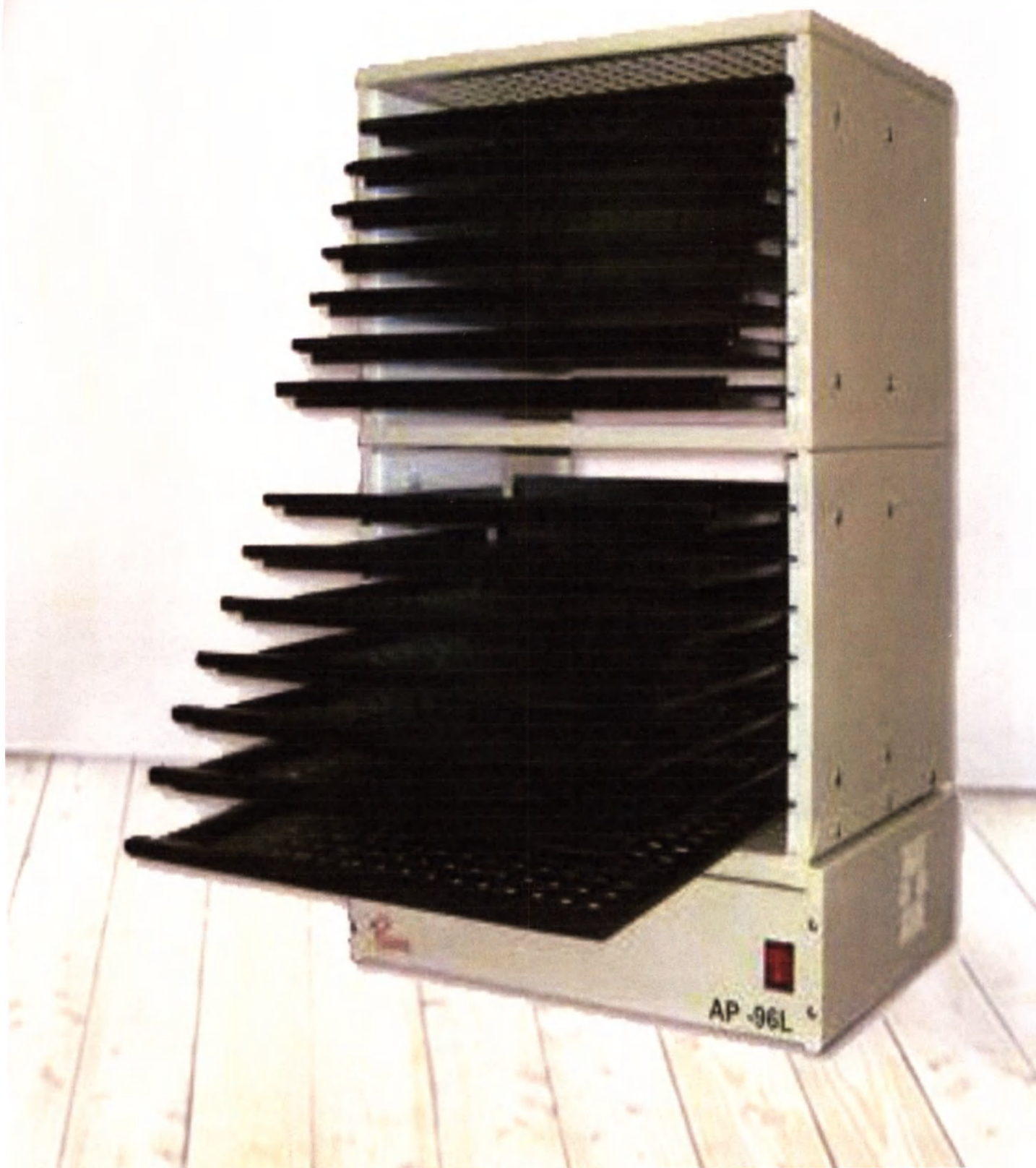
Общий вид перемешивателя тромбоцитов AP-96L
