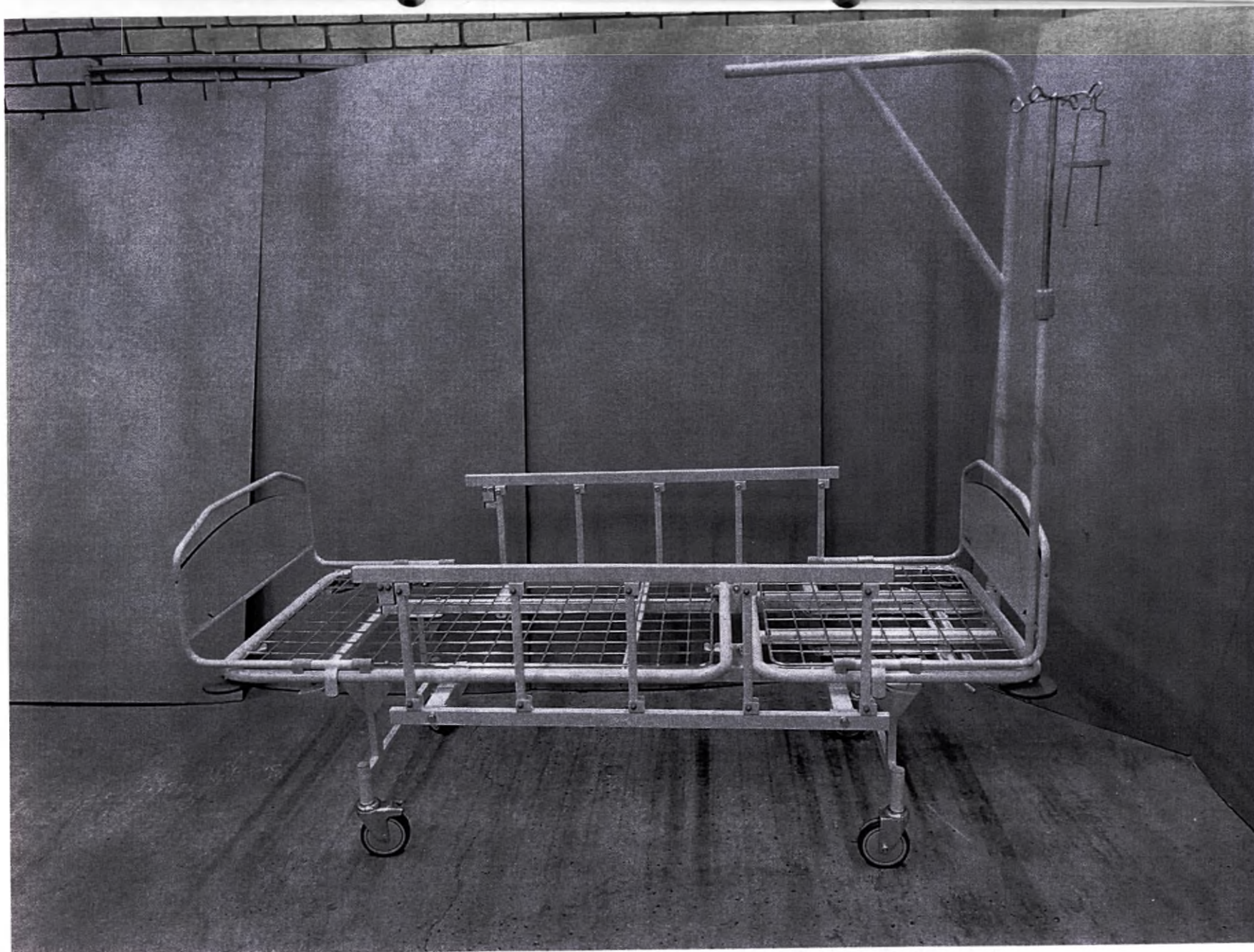
«Кровать функциональная КФ-2 - «Айболит» ТУ 9452-010-51768895-2004 Общий вид с принадлежностями
