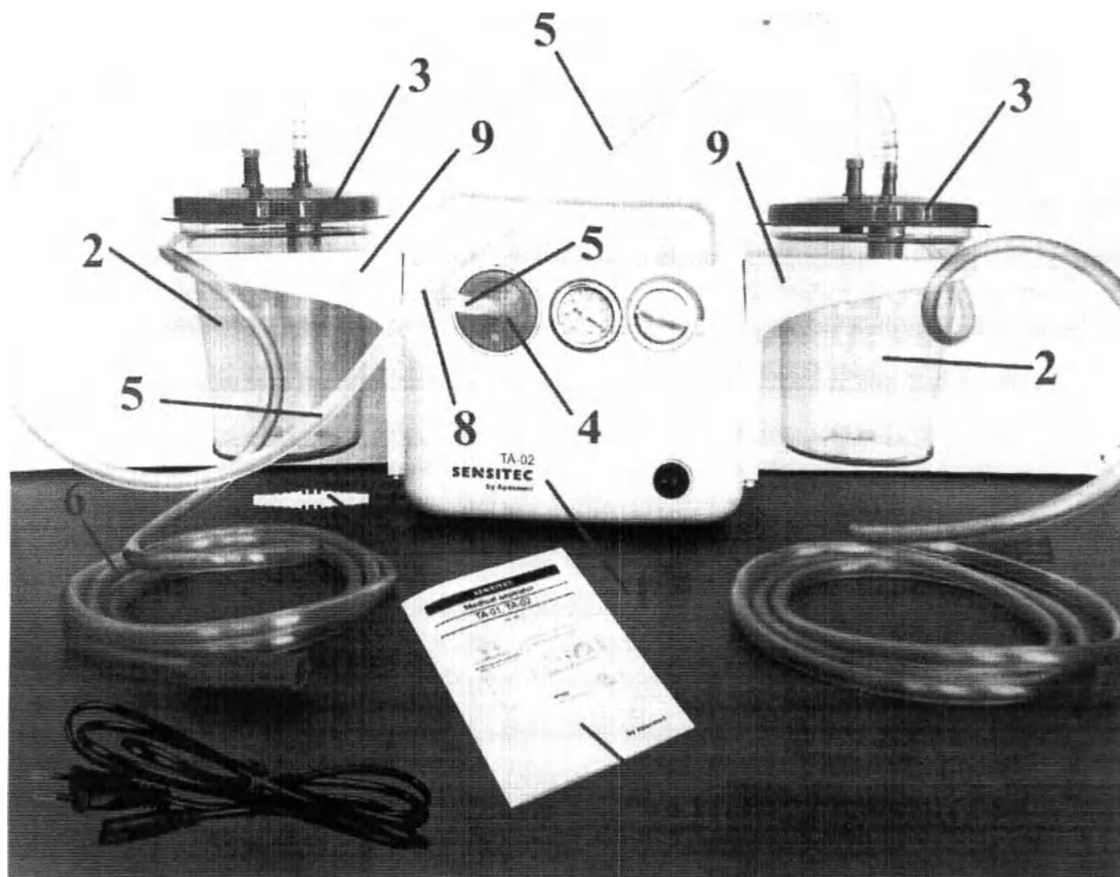
Аспиратор медицинский ТА-02 в составе:
