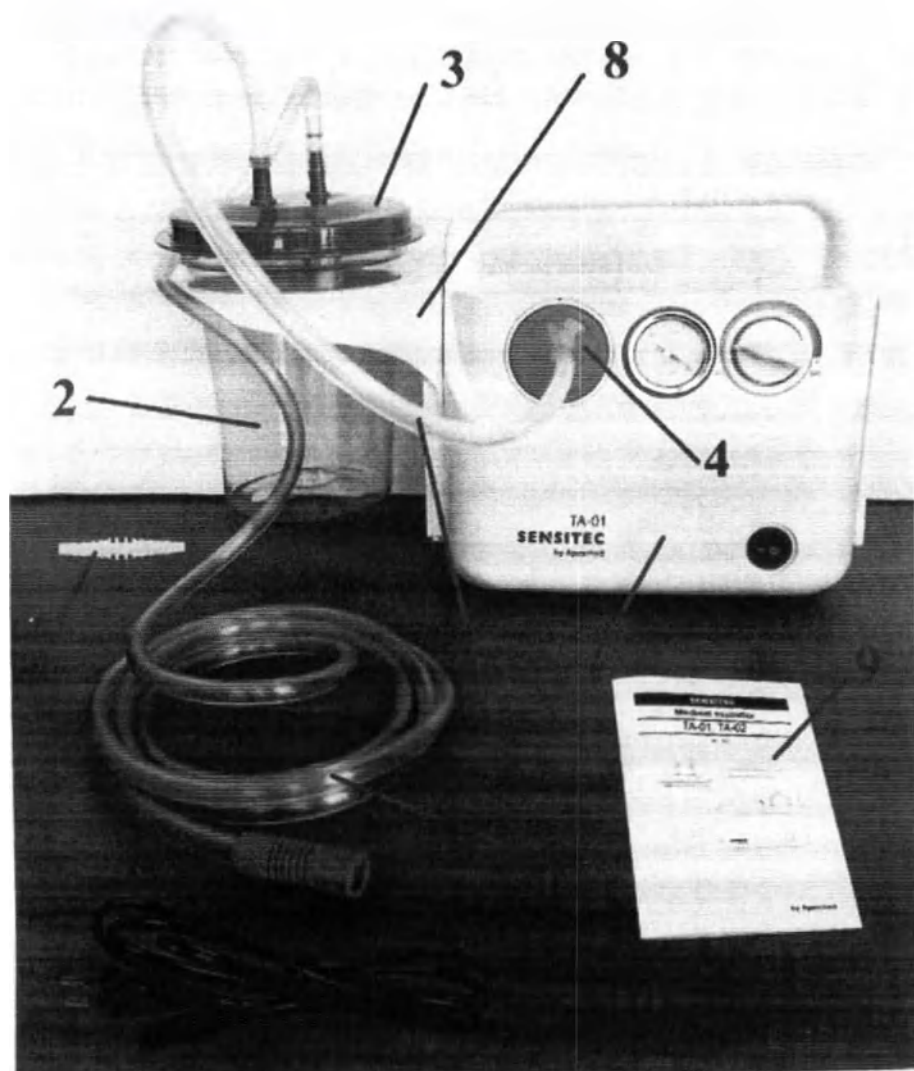
Аспиратор медицинский ТА-01 в составе:
