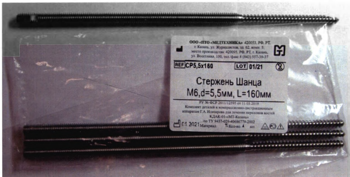
Стержень Шанца, M6, d=6,0мм, L=160мм (CP5,5x160)
