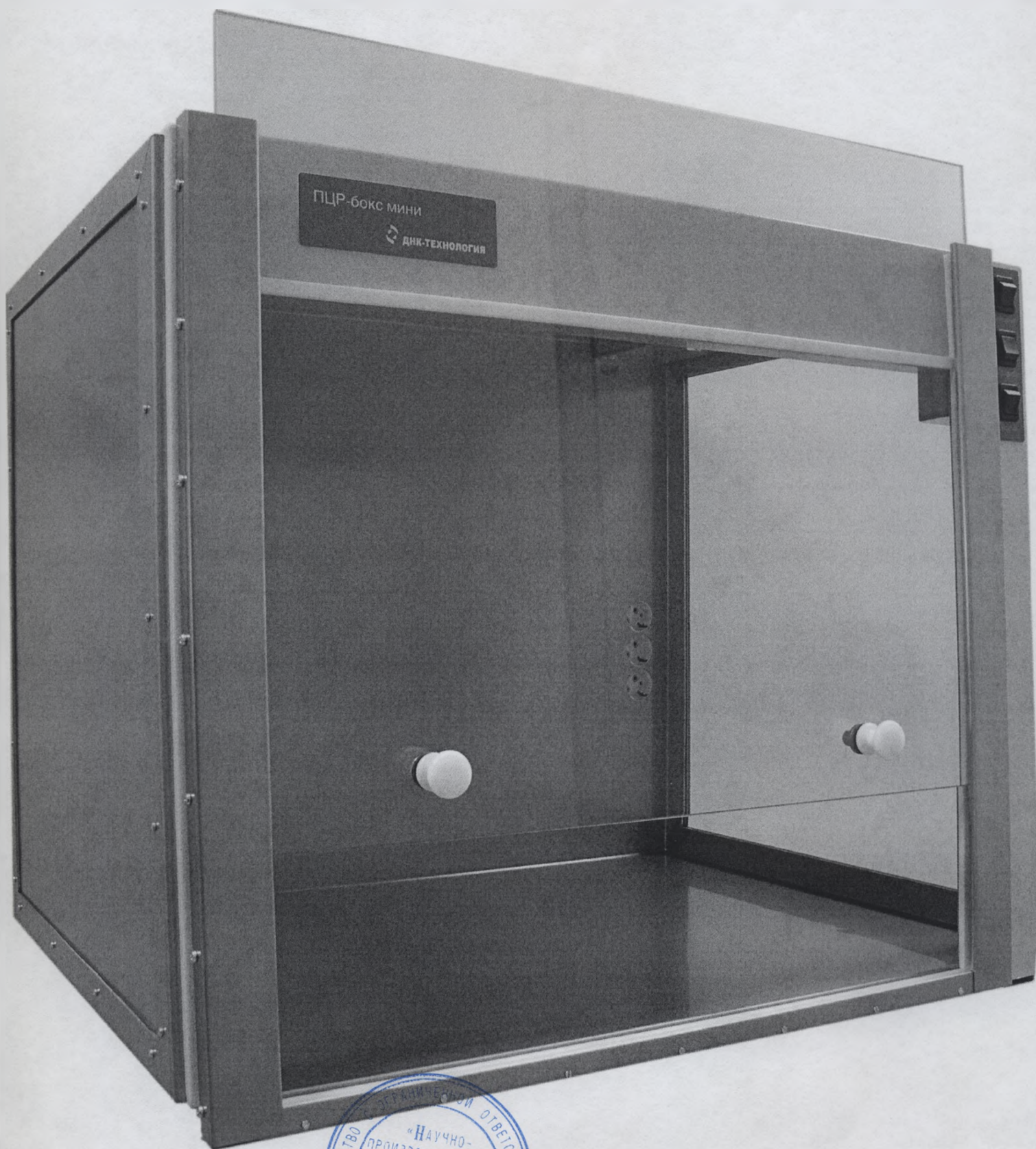
Фото ПЦР-Бокс мини
