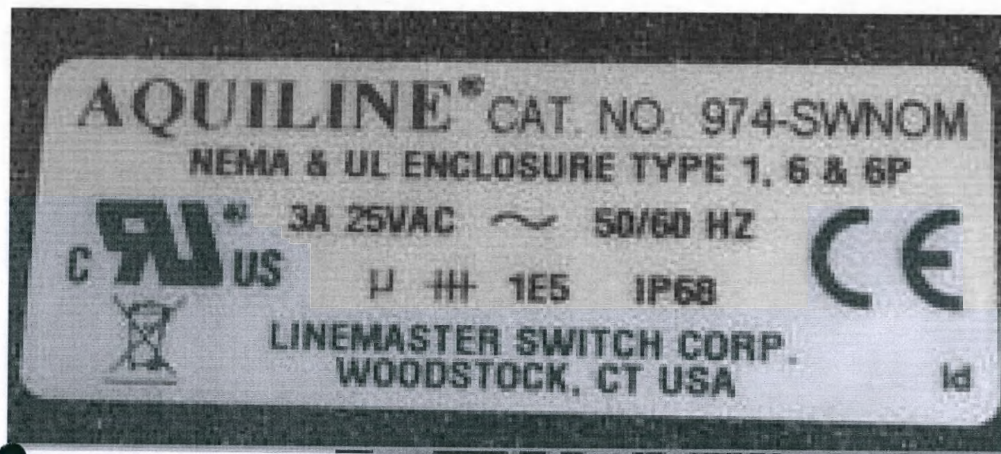
Рисунок 16.1. Маркировка ножной педали
