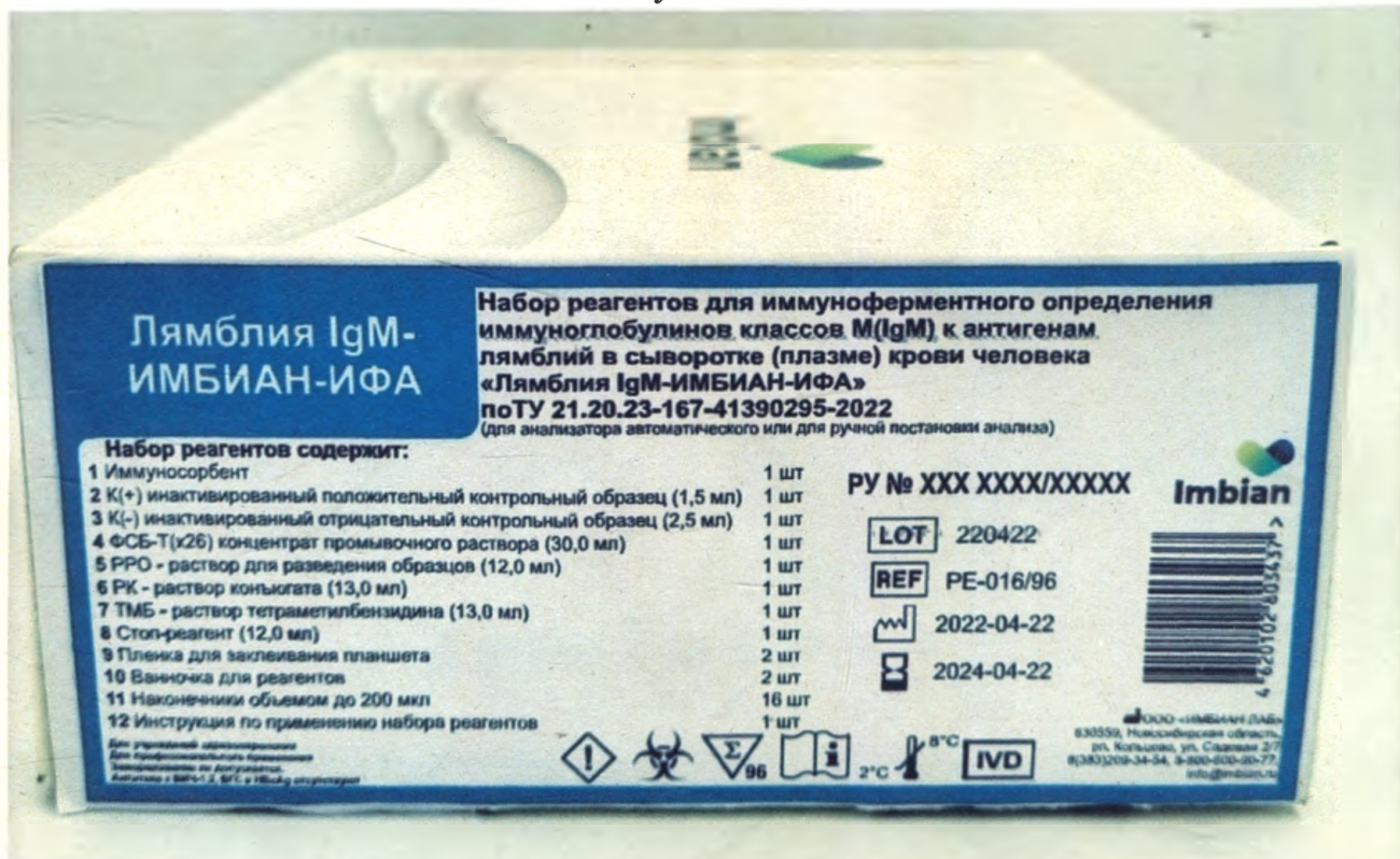
Фото упаковки
