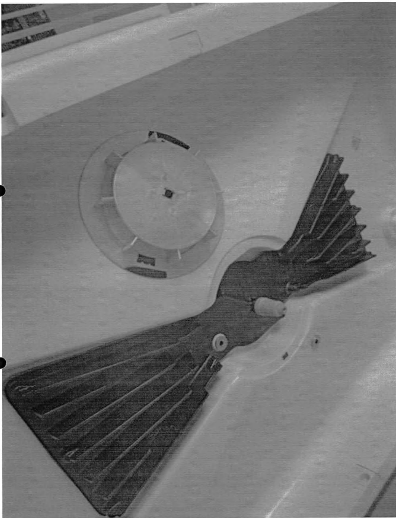
26. Вентилятор для циркуляции воздуха.
