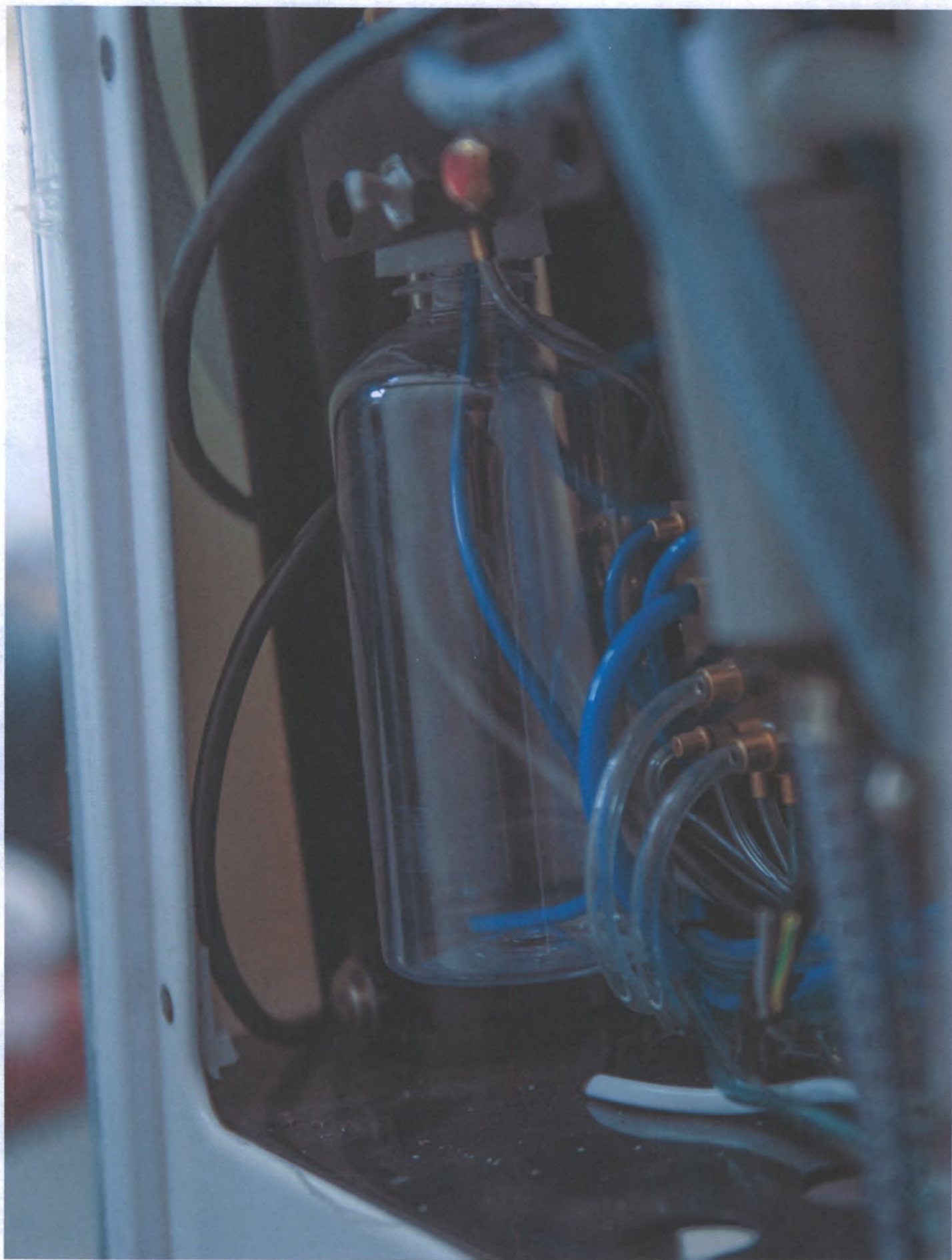
Гидроблок для моделей X5, X5 + X5 + cart: бутылка для воды и дезинфицирующей жидкости для установки внутри корпуса гидроблока
