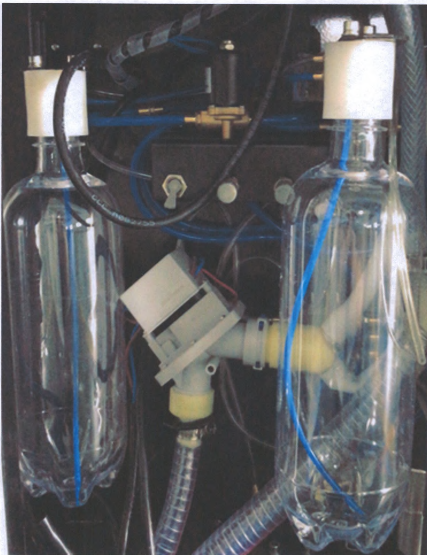
Гидроблок X5 +Floor: бутылка для воды и дезинфицирующей жидкости для установки внутри корпуса гидроблока
