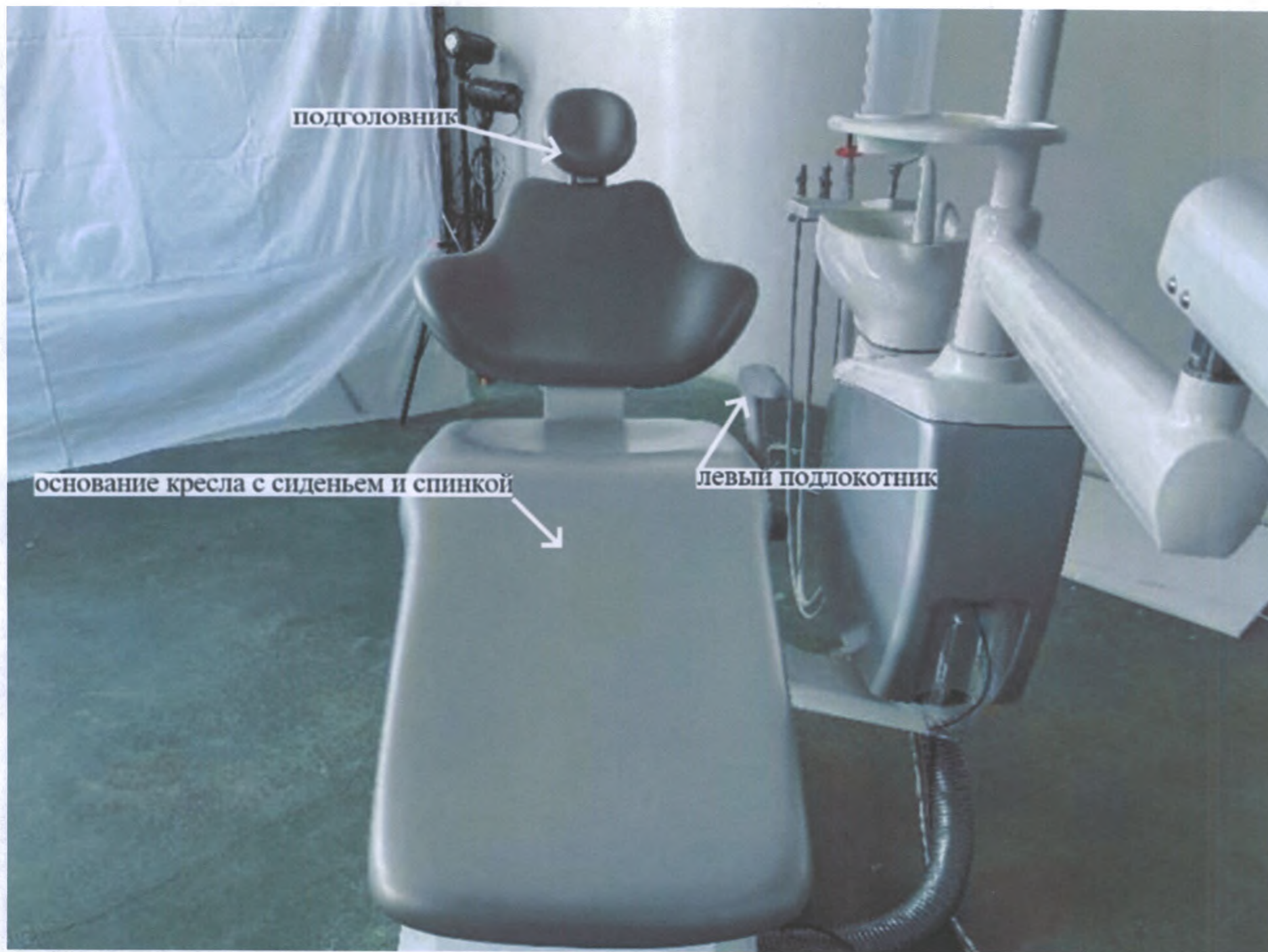
Кресло стоматологическое для серии X1, в составе: основание кресла с сиденьем и спинкой, левый подлокотник, подголовник
