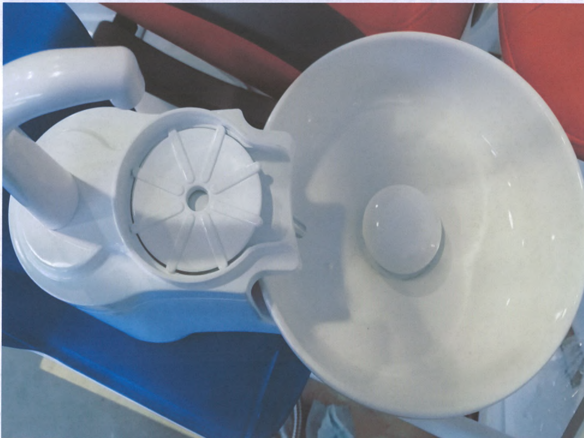
Чаша пловательницы керамическая для серии X5 с канюлями наполнения стакана и промыва чаши и двумя съемными фильтрами-ловушкой
