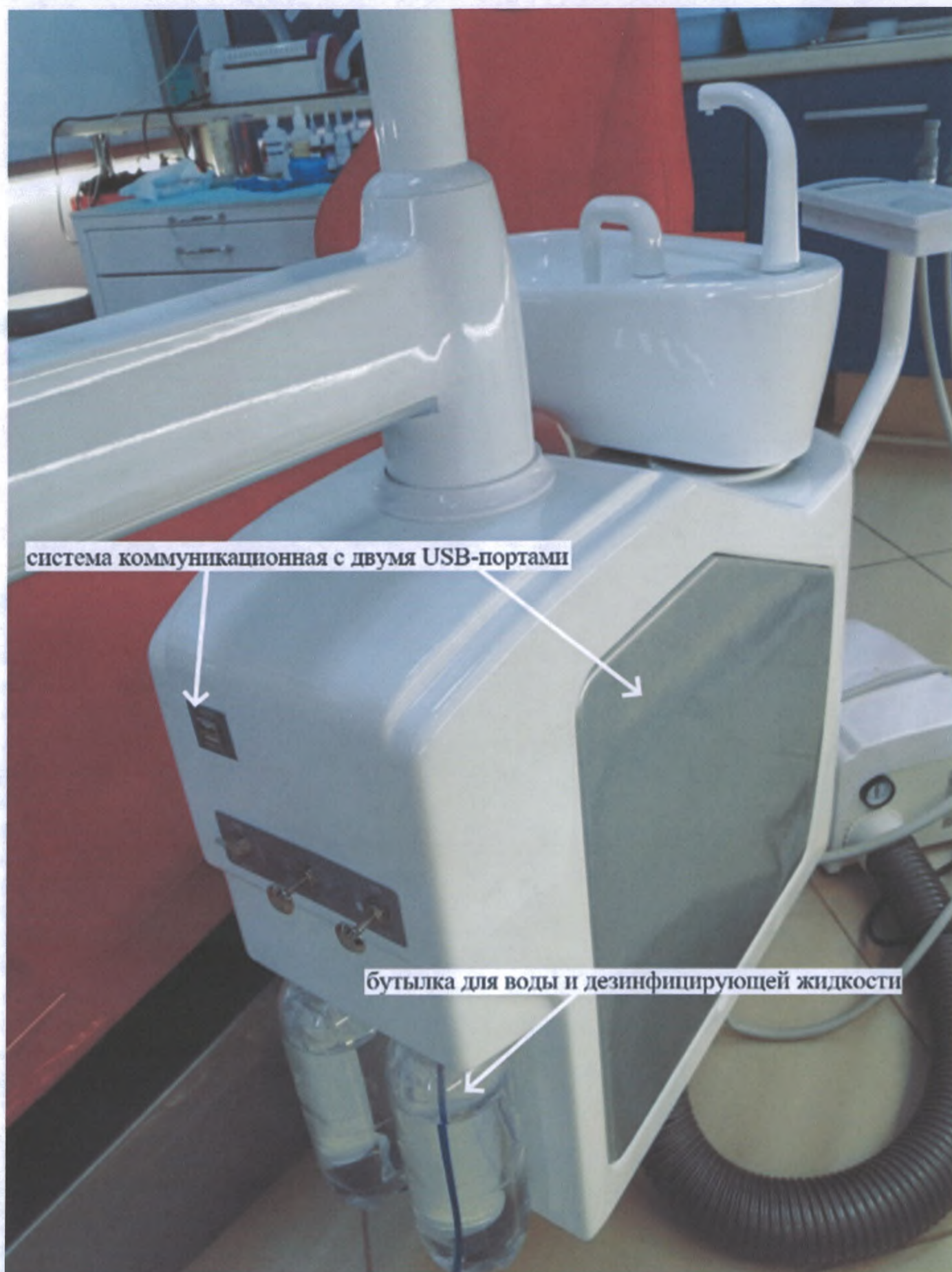
Гидроблок для серии X3: система коммуникационная с двумя USB-портами, бутылка для воды и дезинфицирующей жидкости
