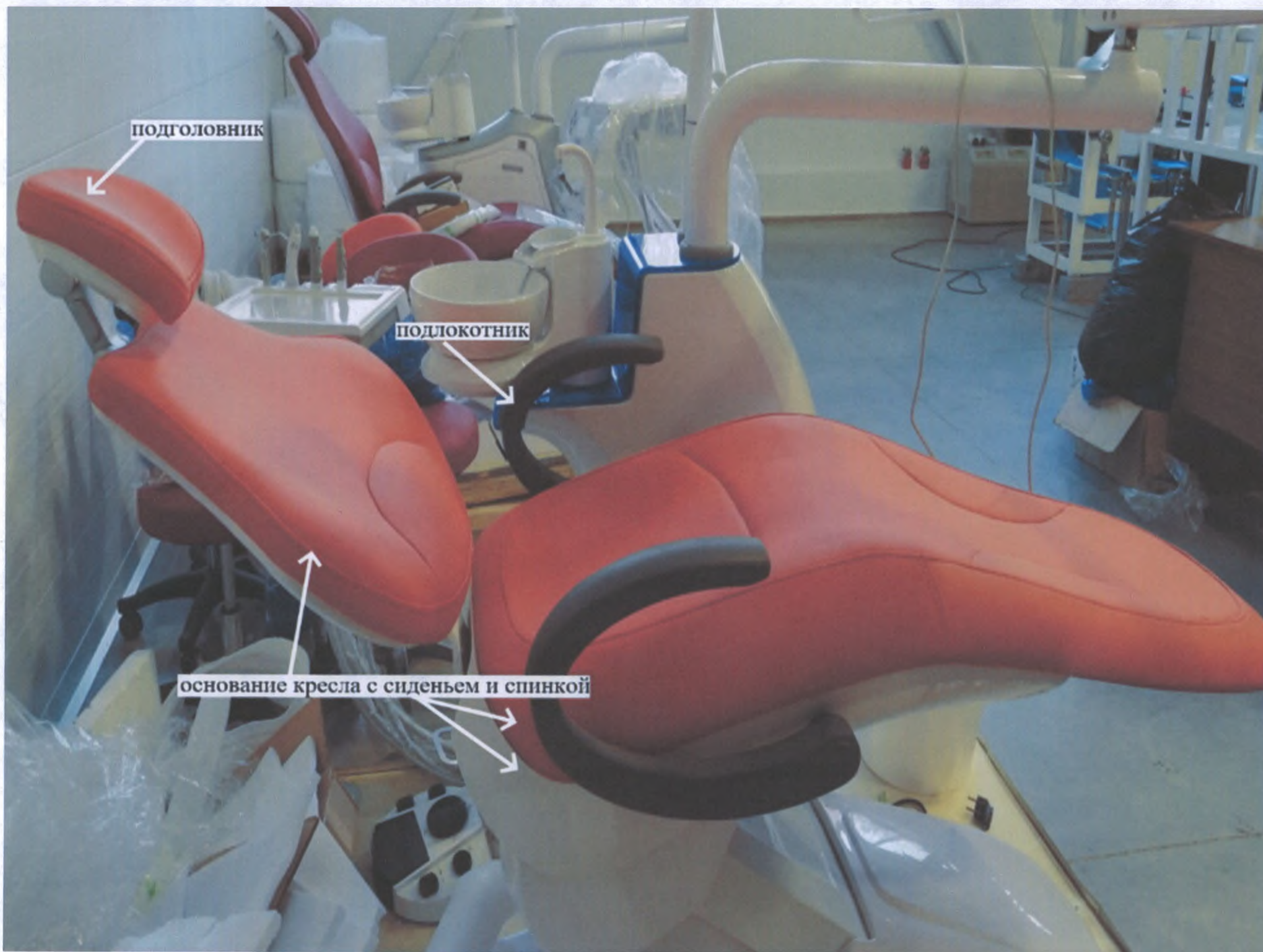
Кресло стоматологическое для серии X5: основание кресла с сиденьем и спинкой, подлокотник, подголовник
