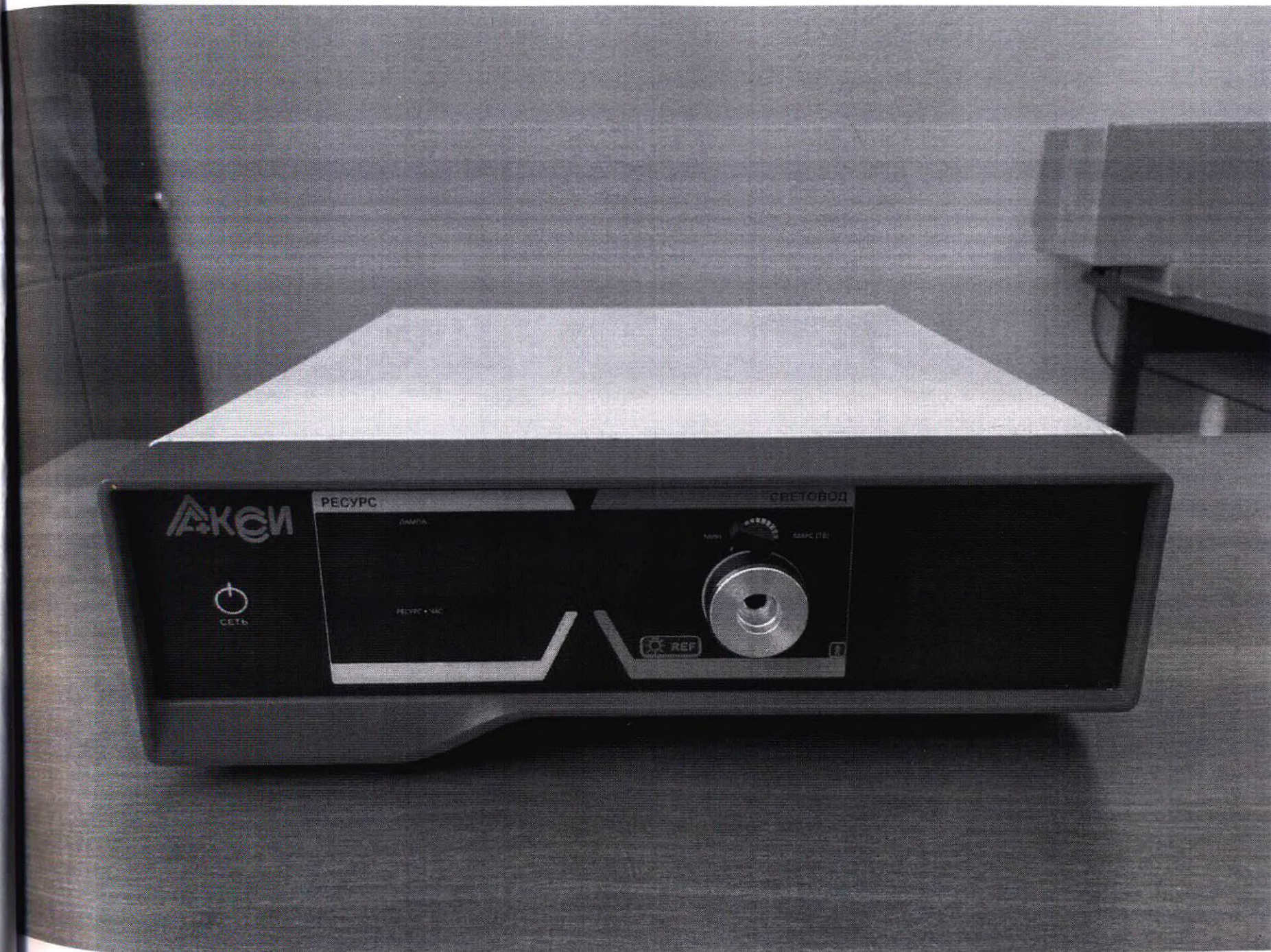
Осветитель эндоскопический с ксеноновым источником света и счетчиком времени его работы для жесткой эндоскопии ООО ЦИРМИ info@cirmi.ru www.goszdravnadzor.ru ОЭКГМ – «АКСИ» тип 2
