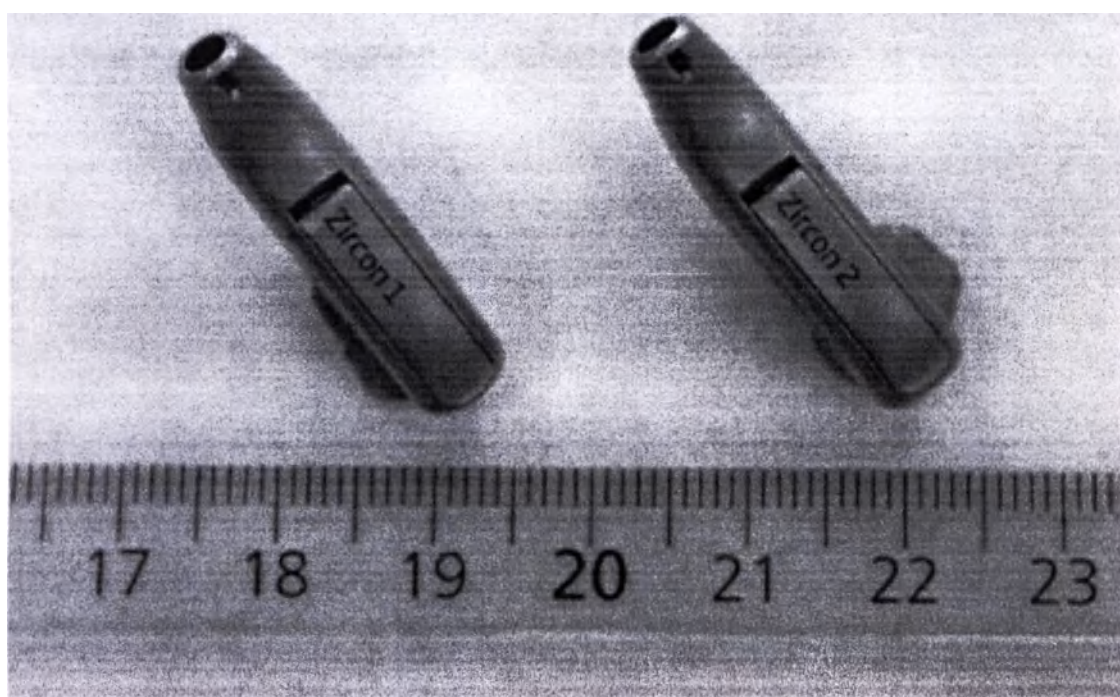
Аппарат слуховой воздушной проводимости с приемником в ухе ZIRCON 1, MINIRITE T Аппарат слуховой воздушной проводимости с приемником в ухе ZIRCON 2, MINIRITE T
