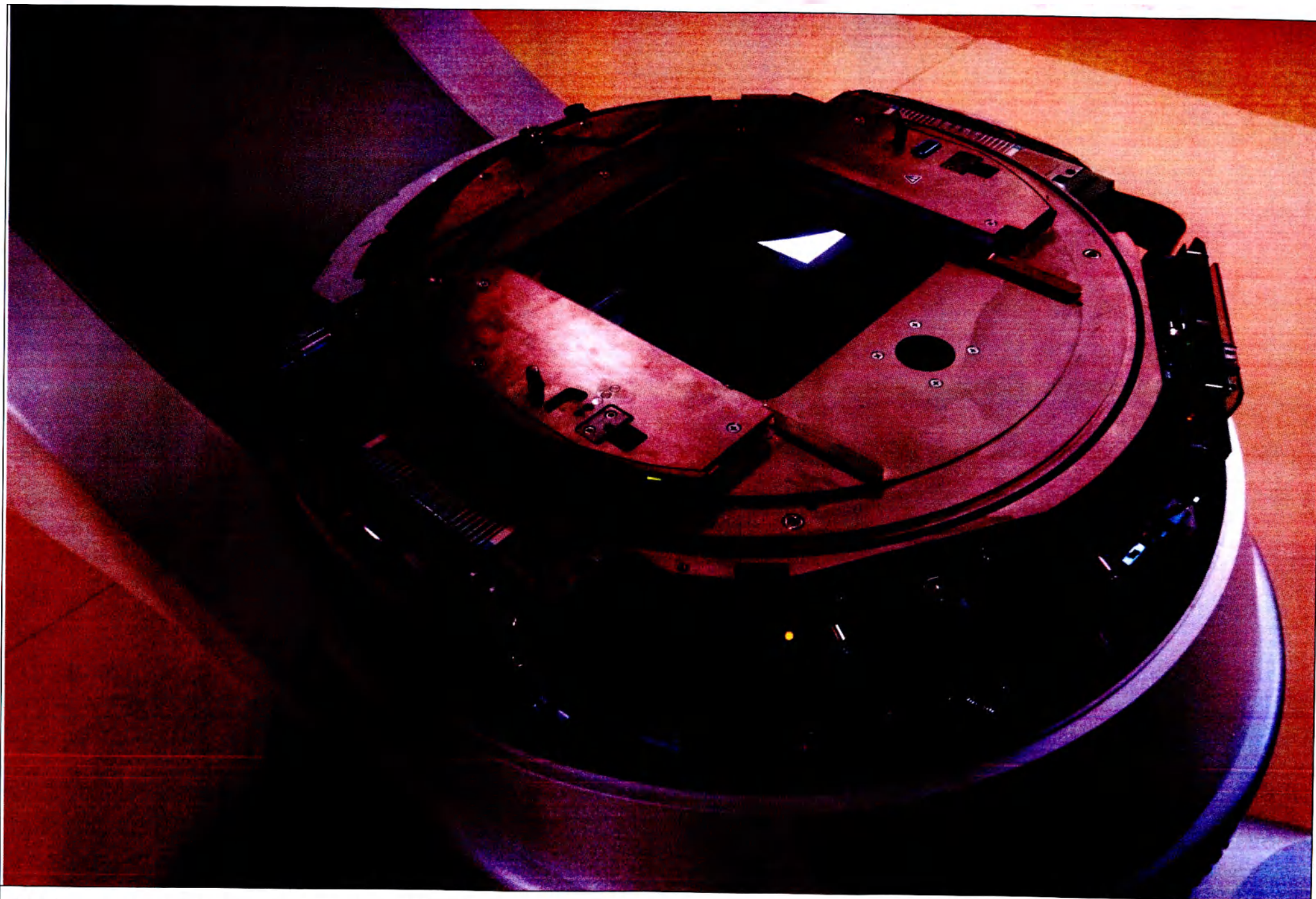
56. Многолепестковый коллиматор 120 или 120HD.
