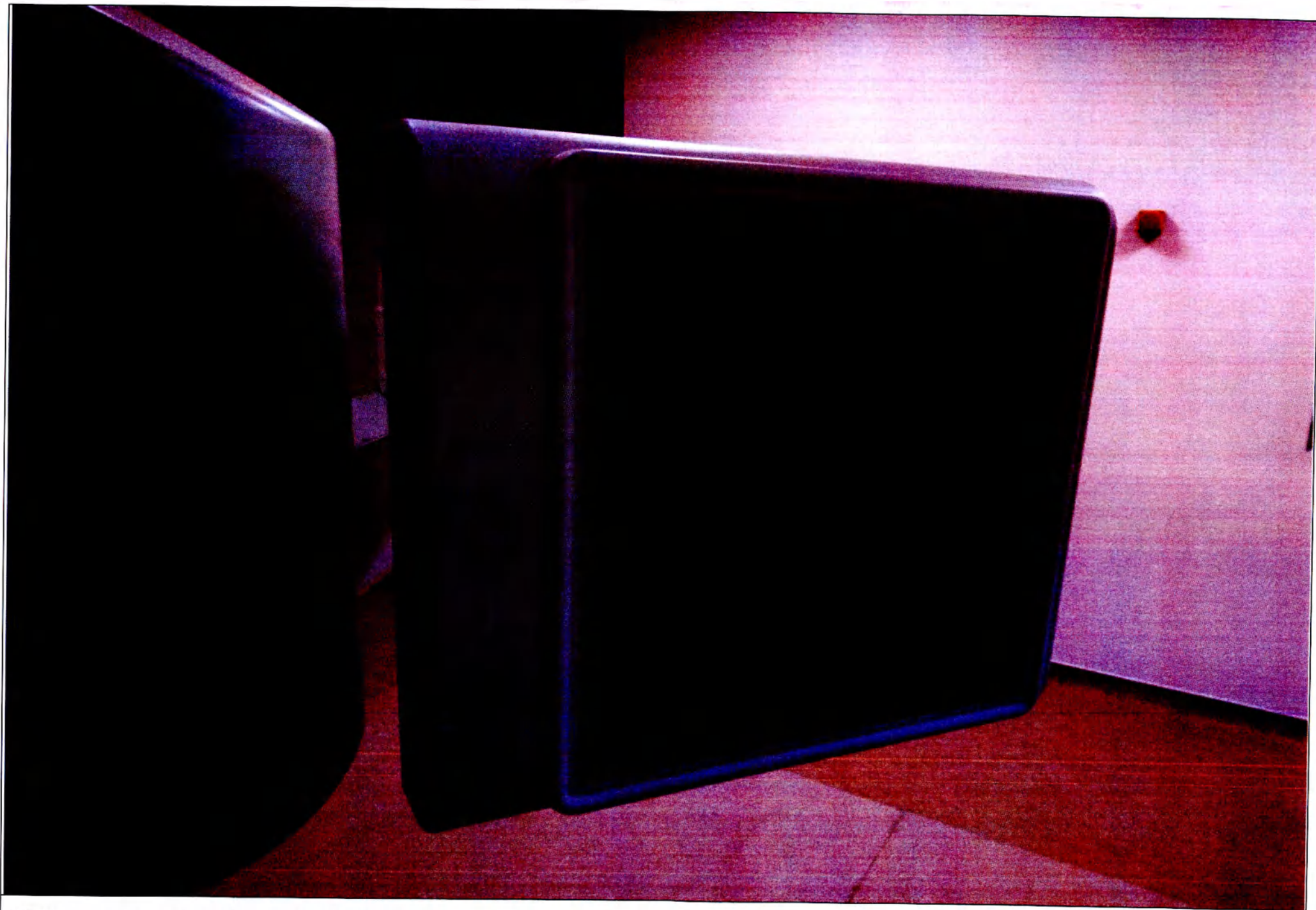
76. Встроенная система рентгеновизуализации.
