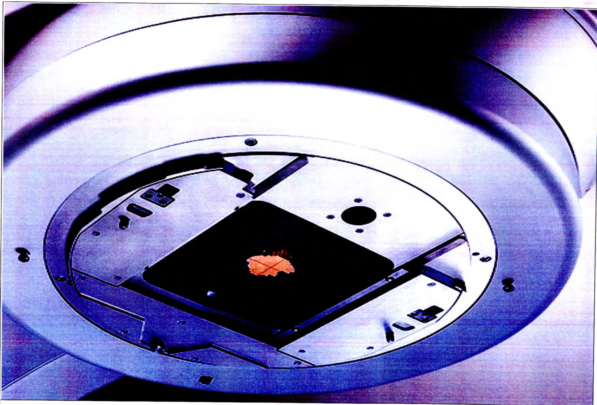
5а. Многолепестковый коллиматор 120 или 120HD.
