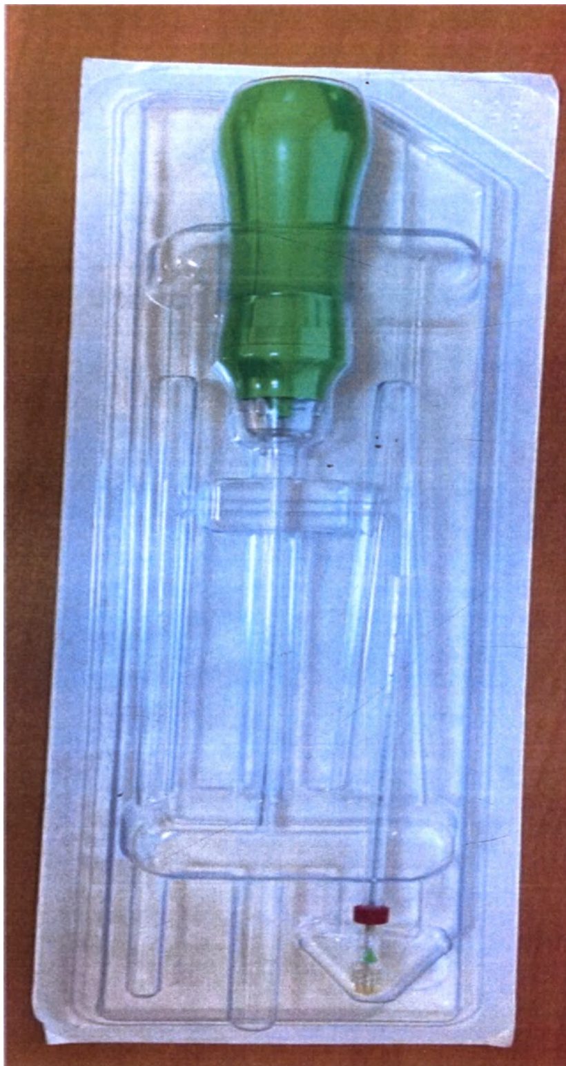
Рисунок 3. Внешний вид изделия в стерильной упаковке: первичная упаковка блистер с крышкой вариант исполнения, артикул DKR1716CDFL10(17G) – красный ограничитель
