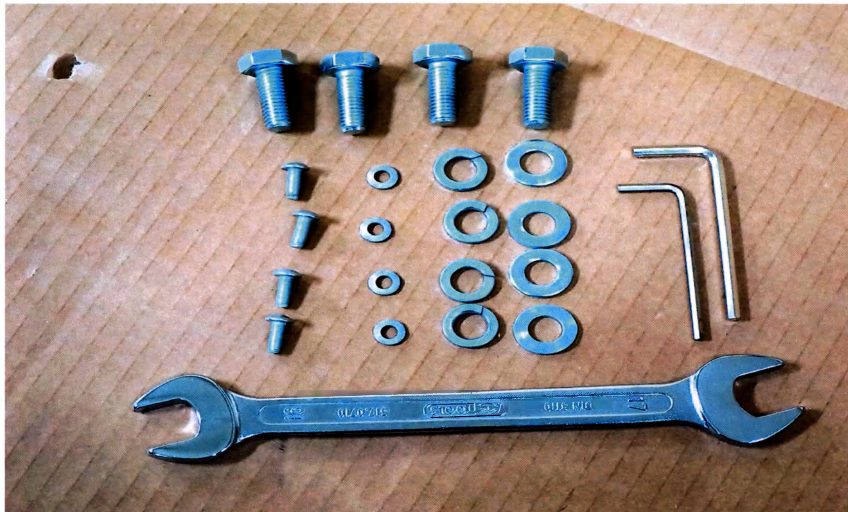
Рис. 6 Крепёж сборочный: болт 10x25 мм - 4 шт. (1), винт 5x12 мм - 4 шт.(2), шайба 10x10 мм - 4 шт.(3), шайба гроверная x10 мм (4), шайба гроверная 5x10 мм - 4 шт.(5), ключ шестигранный торцевой x3 мм (6), ключ шестигранный торцевой x4 мм (7), ключ рожковый x 17 мм (8)
