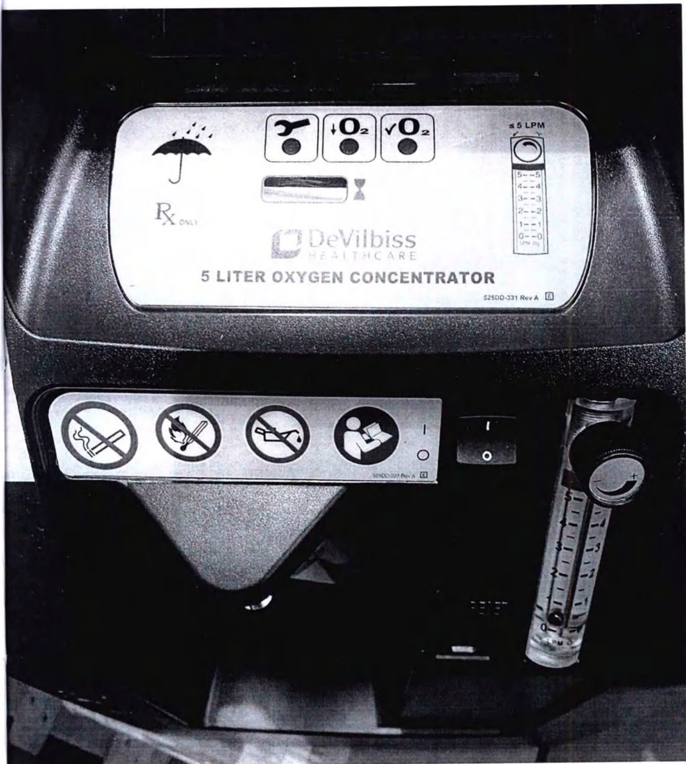
Концентратор кислорода «DeVilbiss» 525, 5 литров (артикул 525KS) – передняя панель
