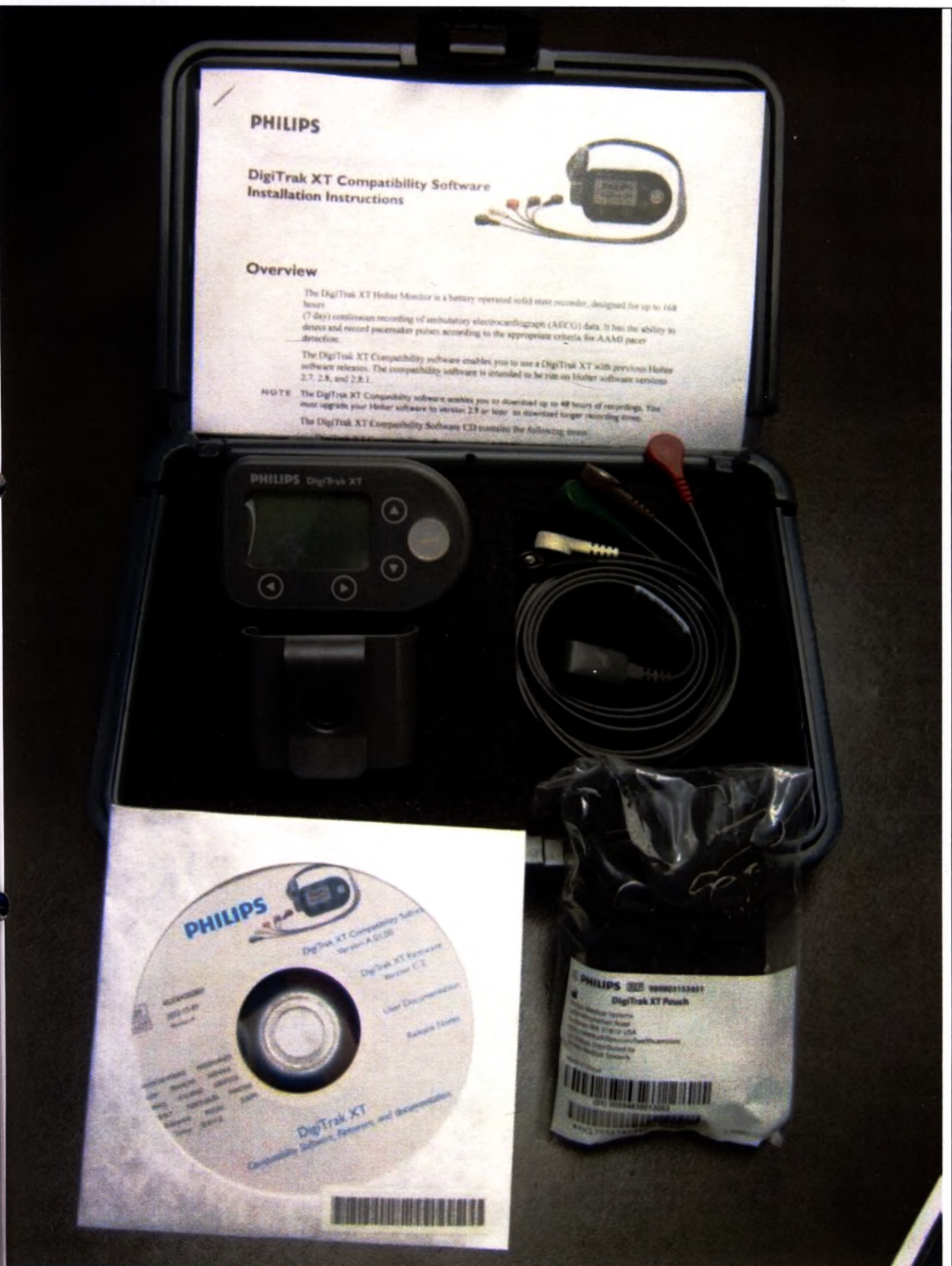
1.2. Монитор холтеровский DigiTrak XT с принадлежностями. Общий вид в упаковке.
