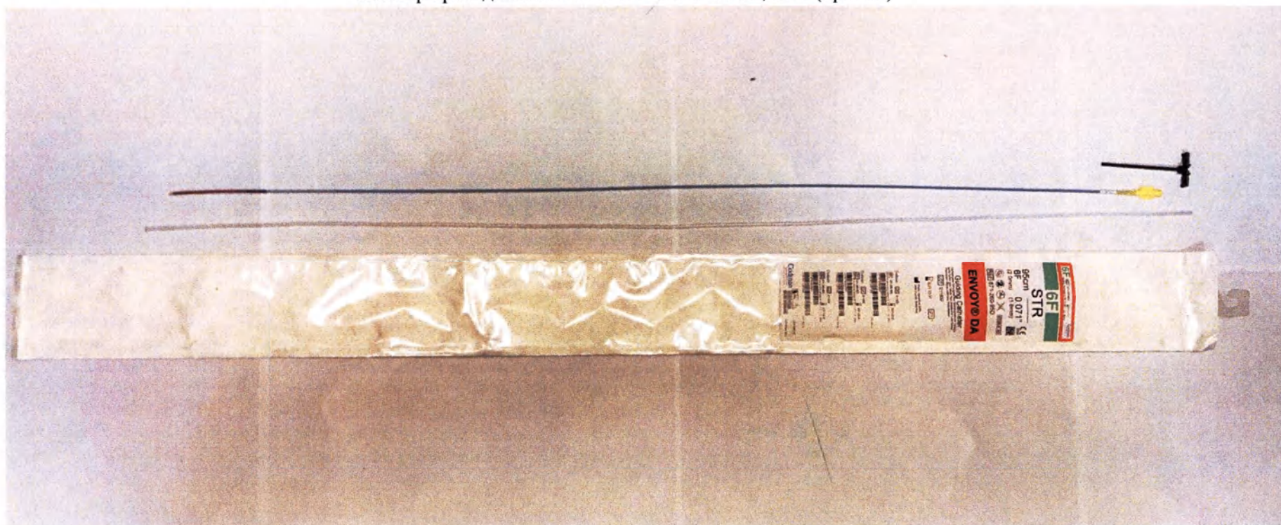
Катетер проводниковый ENVOY DA 6F 95 см, STR (прямой)
