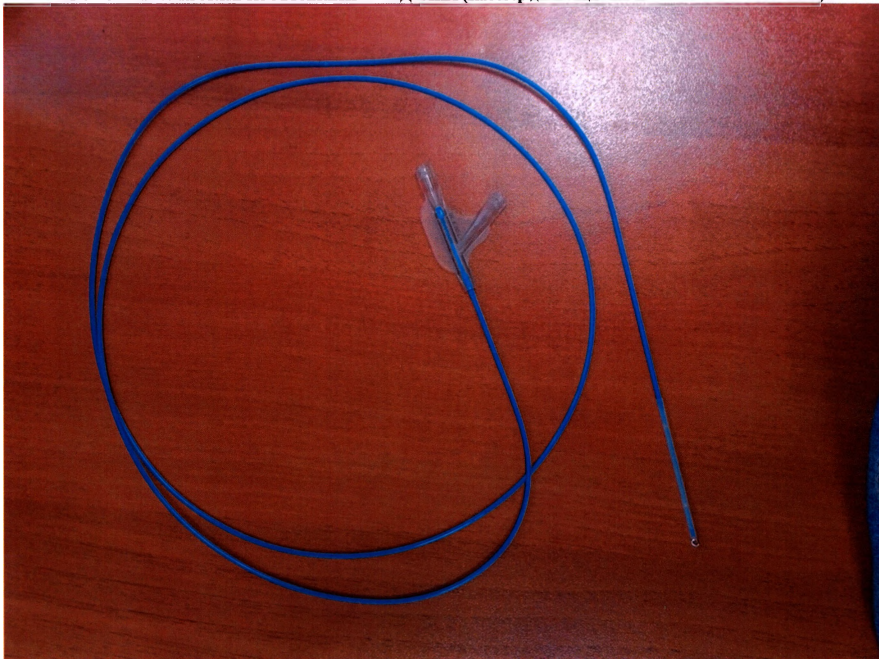
Рис 1. Катетер дилатационный баллонный Mozec PTA
