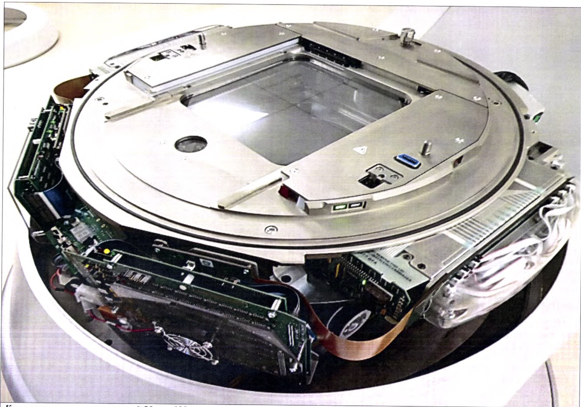
Коллиматор многолепестковый 80 или 120
