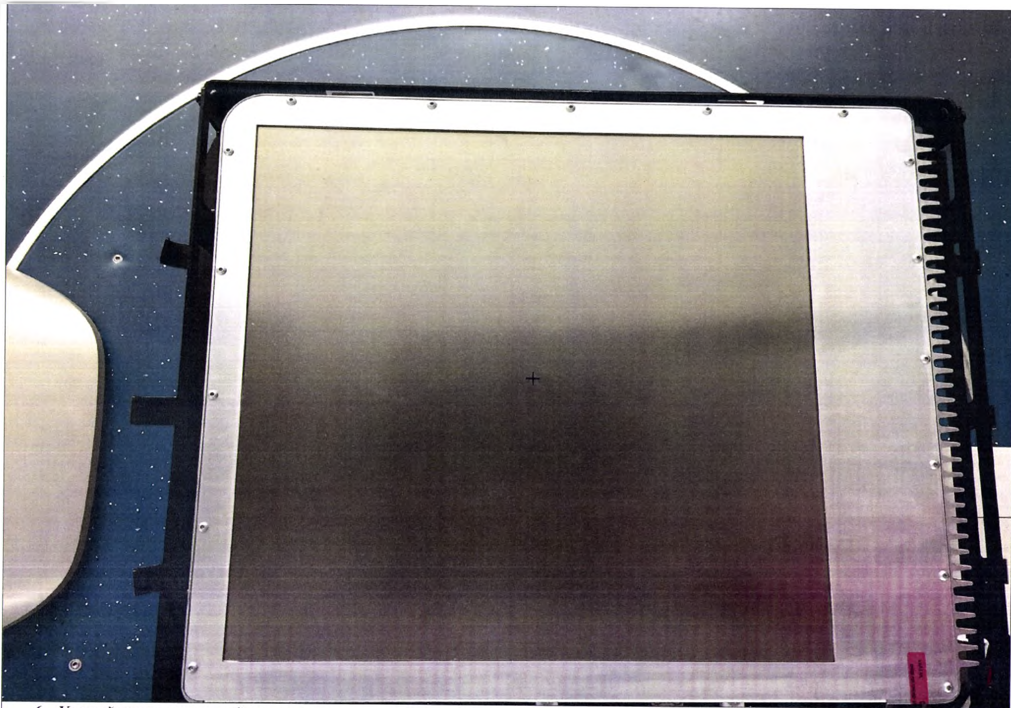
6. Устройство портальной визуализации.
