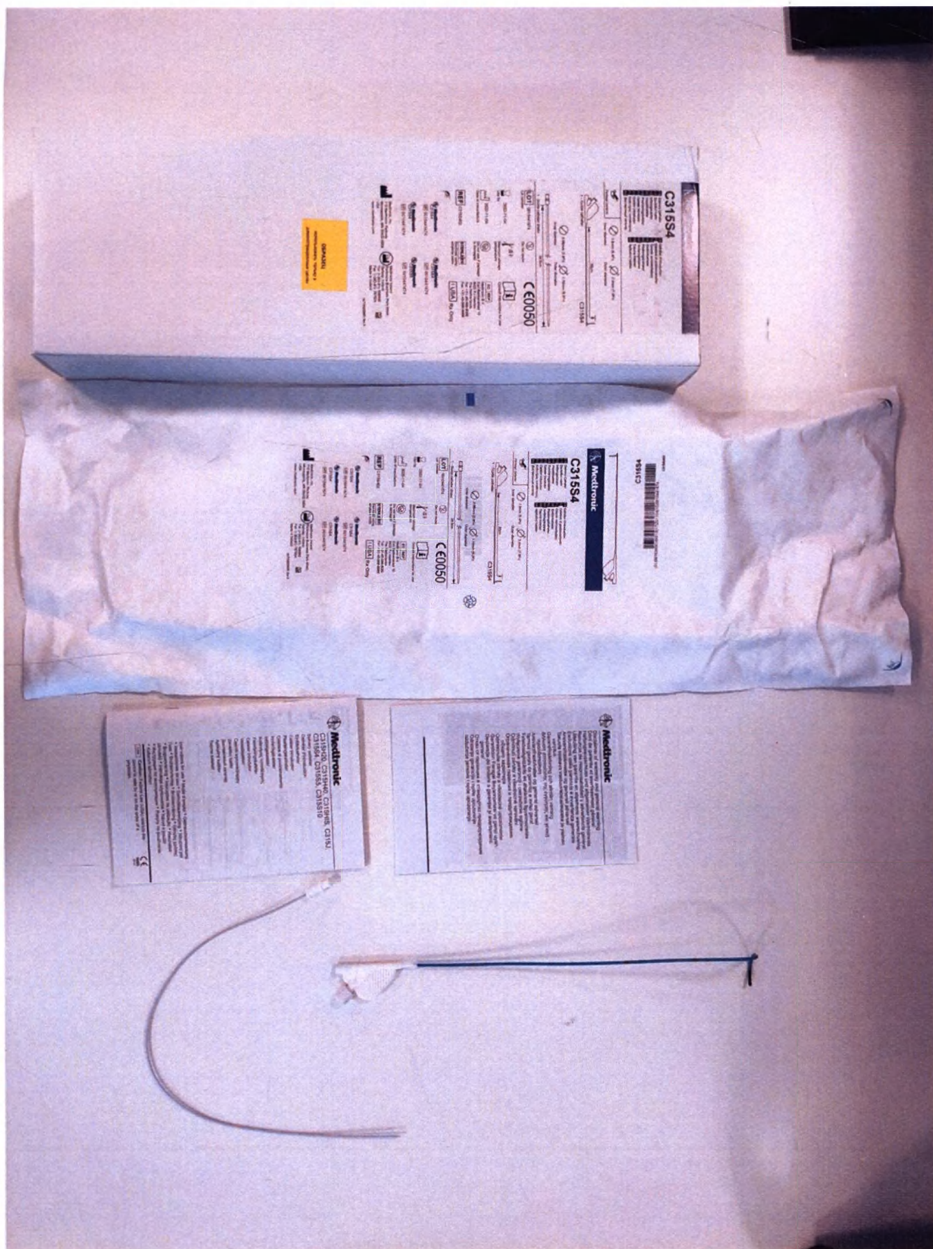
Рисунок 19. Комплект поставки Доставочного катетера (содержимое упаковки) на примере: Доставочного катетера, вариант исполнения: C315S4
