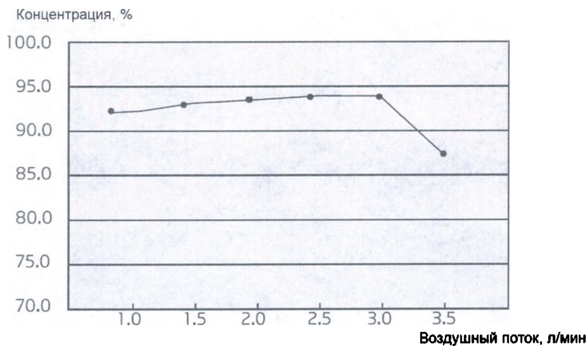
Рис. 75 – График 4 (вариант исполнения 7F-3W (5L))
