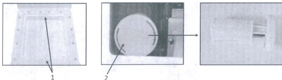
Рис. 50 – Порядок извлечения фильтра тонкой очистки, где:
