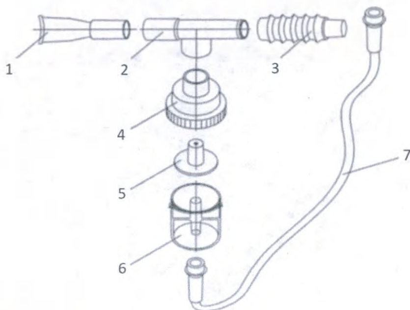
Рис. 70 – Комплект для ингаляции (тип II) (только для 8F-3ZW, 7F-3W (5L), 7F-5BW, 7F-5EW), где:
