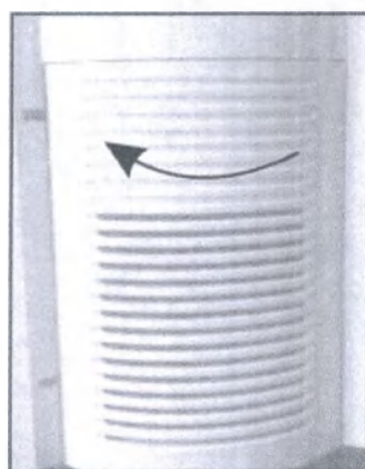
Рис. 63 – Порядок извлечения фильтра грубой очистки
