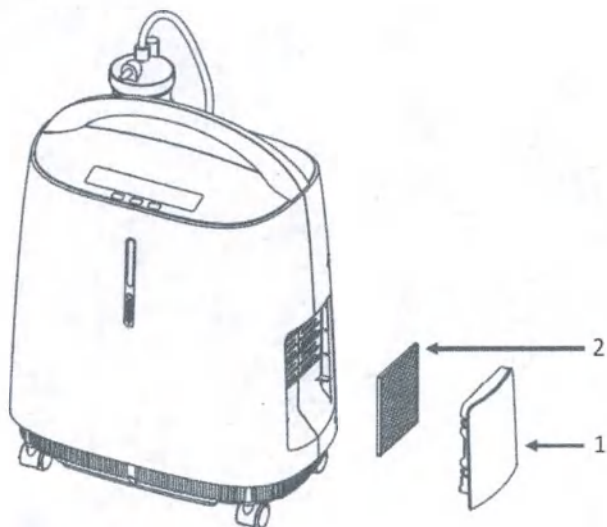
Рис. 29 – Порядок извлечения фильтра, где:
