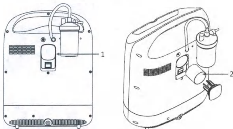
Рис. 36 – Порядок извлечения фильтра тонкой очистки, где:
