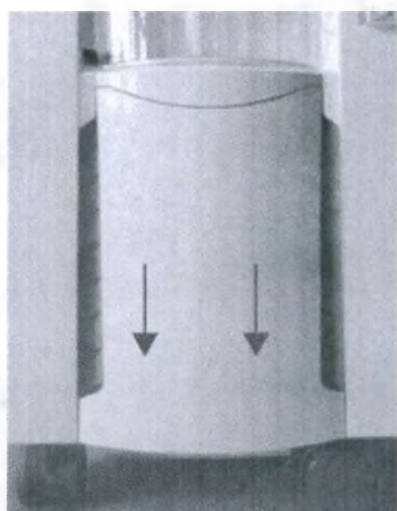
Рис. 56 – Порядок извлечения фильтра грубой очистки
