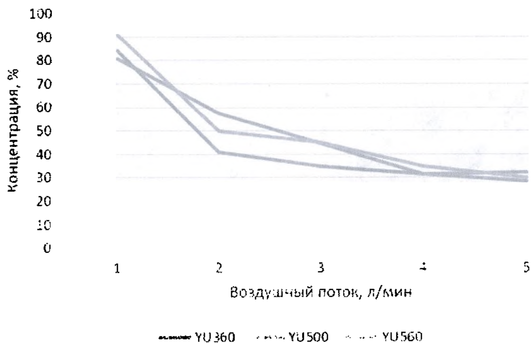
Рис. 72 – График 1 (варианты исполнения YU360, YU500, YU560)
