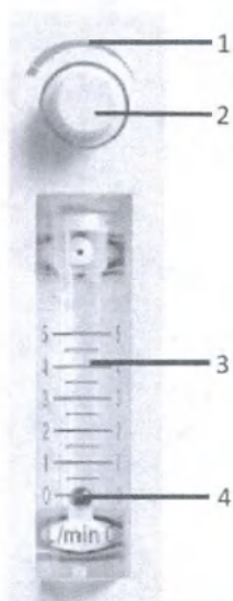
Рис. 54 – Интерфейс скорости потока, где:
