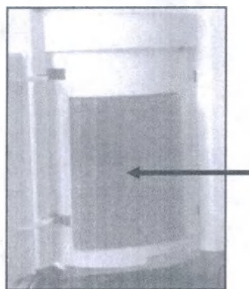
Рис. 62 – Извлечение увлажнителя и место наполнения его водой
