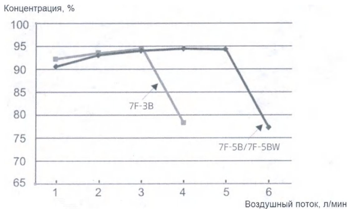
Рис. 74 – График 3 (варианты исполнения 7F-5B, 7F-5BW)
