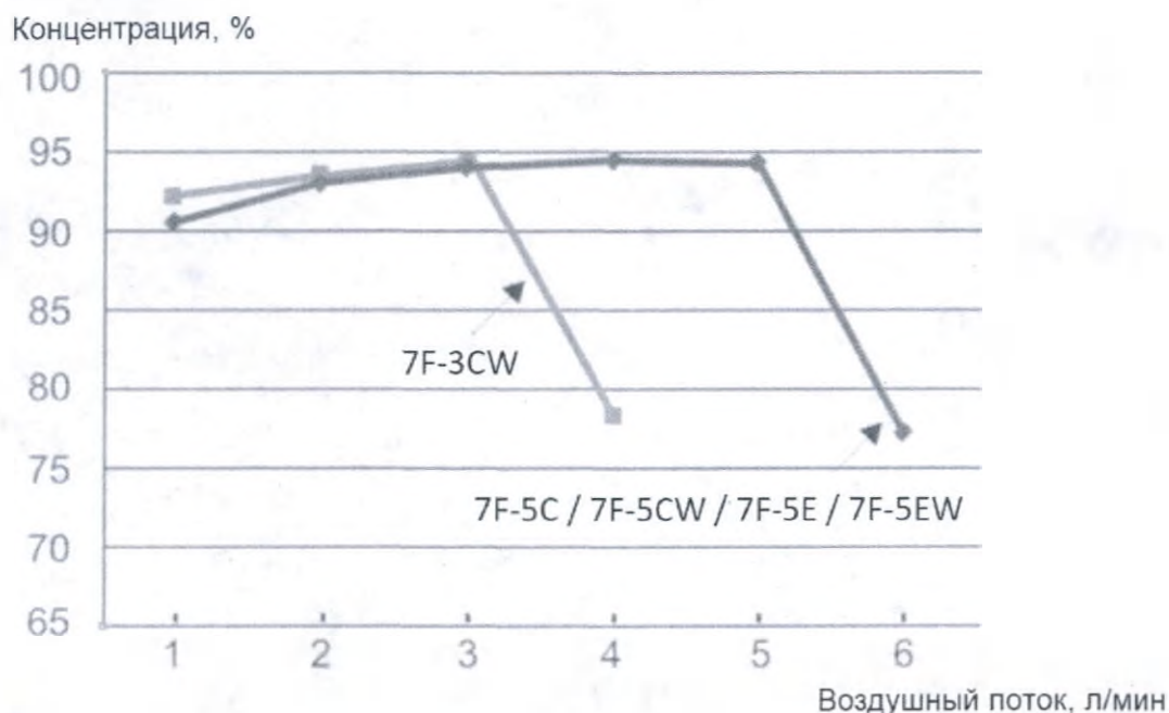
Рис. 76 – График 5 (варианты исполнения 7F-5C, 7F-5CW, 7F-5E, 7F-5EW)
