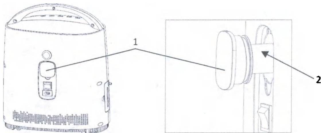
Рис. 14 – Порядок извлечения фильтра тонкой очистки, где:
