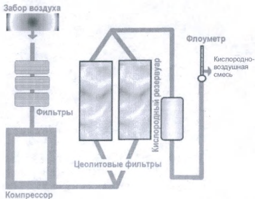
Рис. 71 – Схема, поясняющая процесс получения кислородно-воздушной смеси
