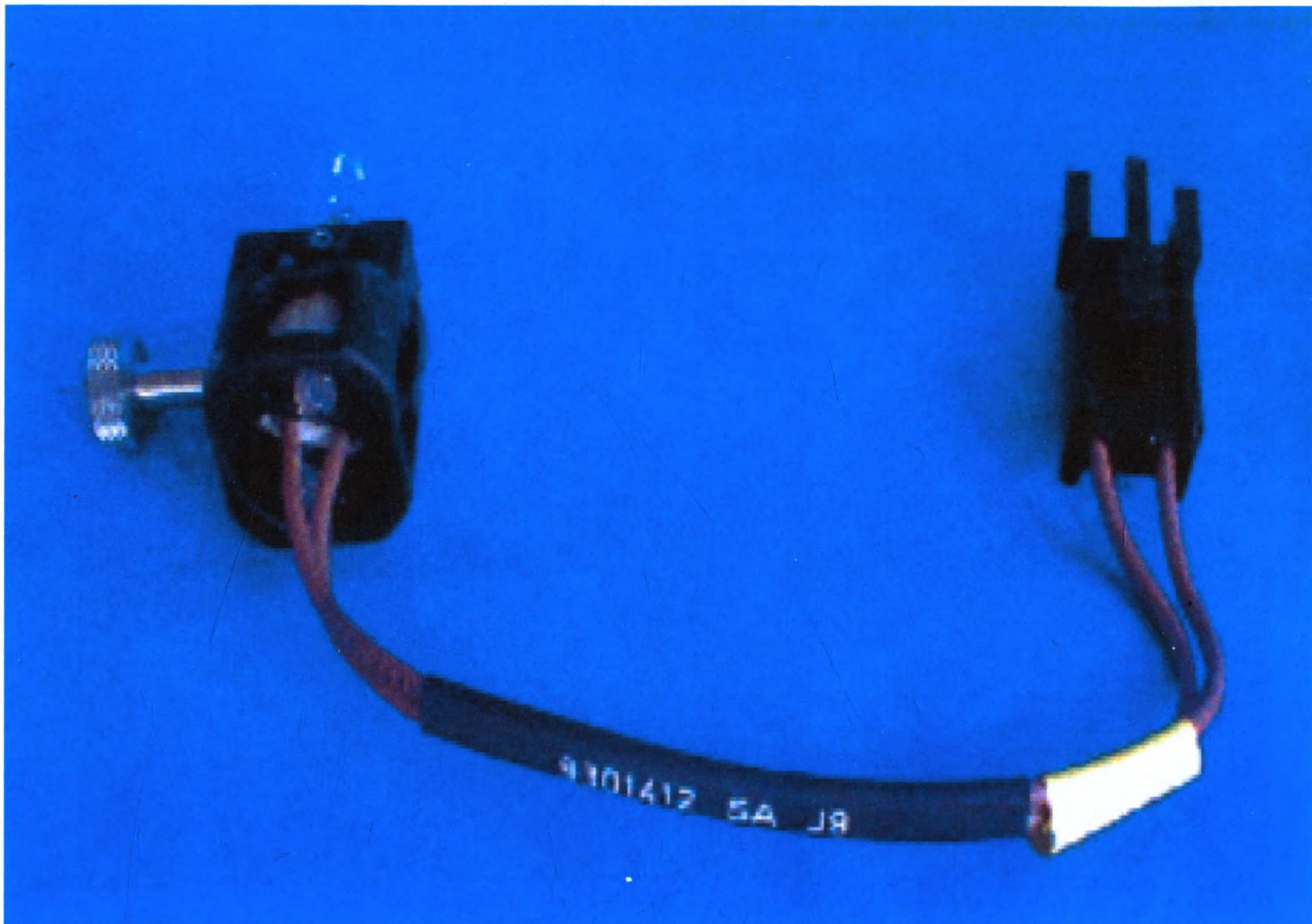
5. Лампа галогеновая 12В/100В в составе с установочным цоколем (Lamp Halogen 12V/100W Assy)
