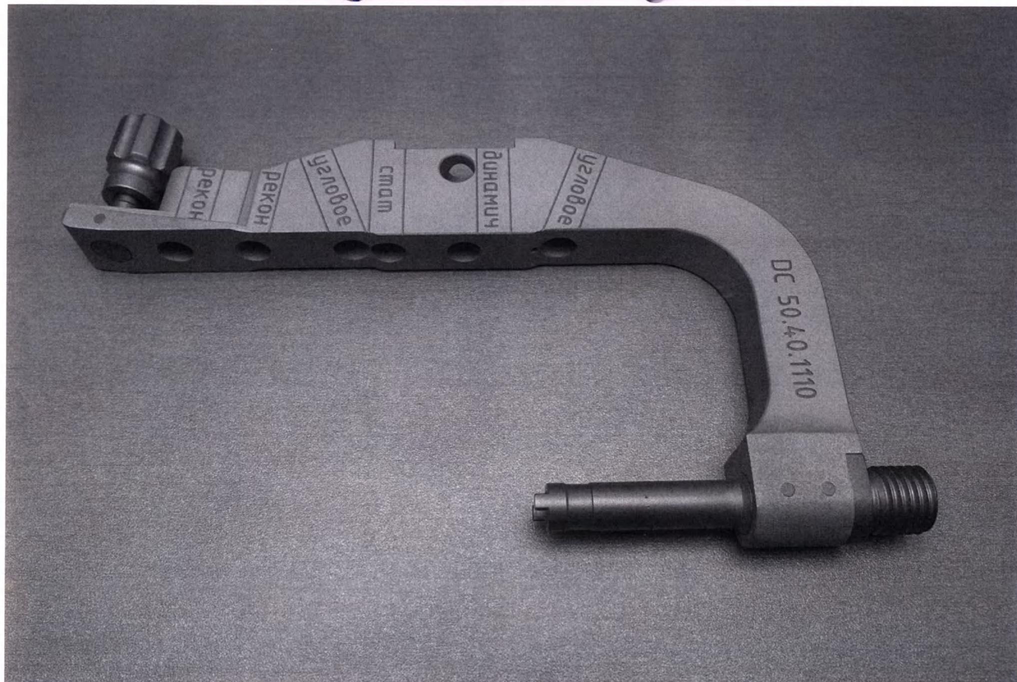
Рисунок 14 - Направитель плечевой на проксимальные отверстия, № 50.40.1110
