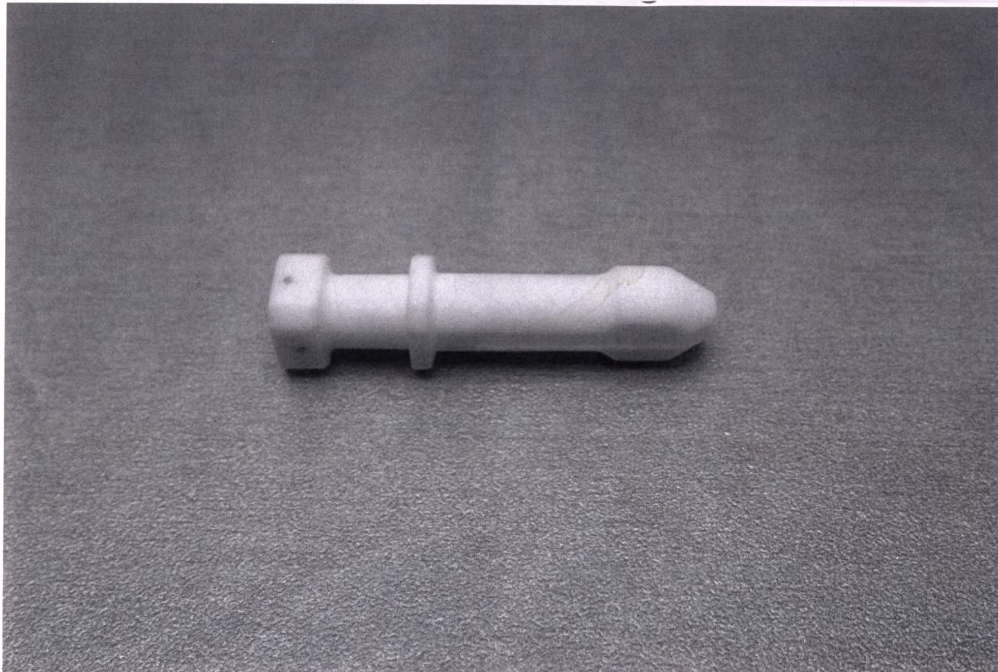
Рисунок 32 - Шаблон-заглушка, № 50.00.9030
