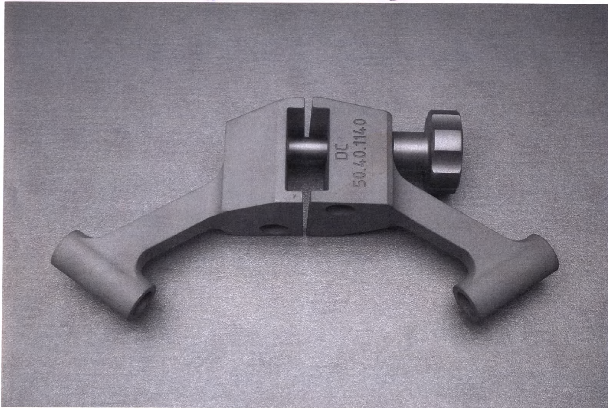
Рисунок 16 - Направитель реконструктивный, № 50.40.1140
