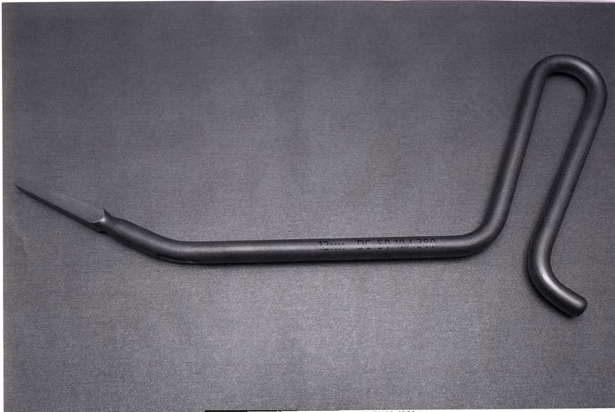
Рисунок 33 - Шило канюлированное, № 50.10.4380
