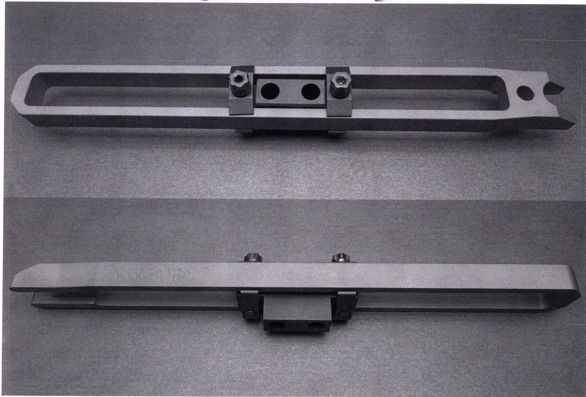
Рисунок 15 - Направитель дистальный, № 50.40.1120
