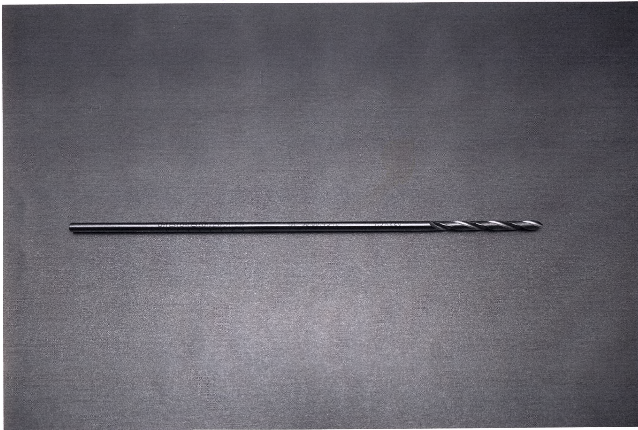
Рисунок 28 - Сверло с измерительной шкалой, № 50.00.4340
