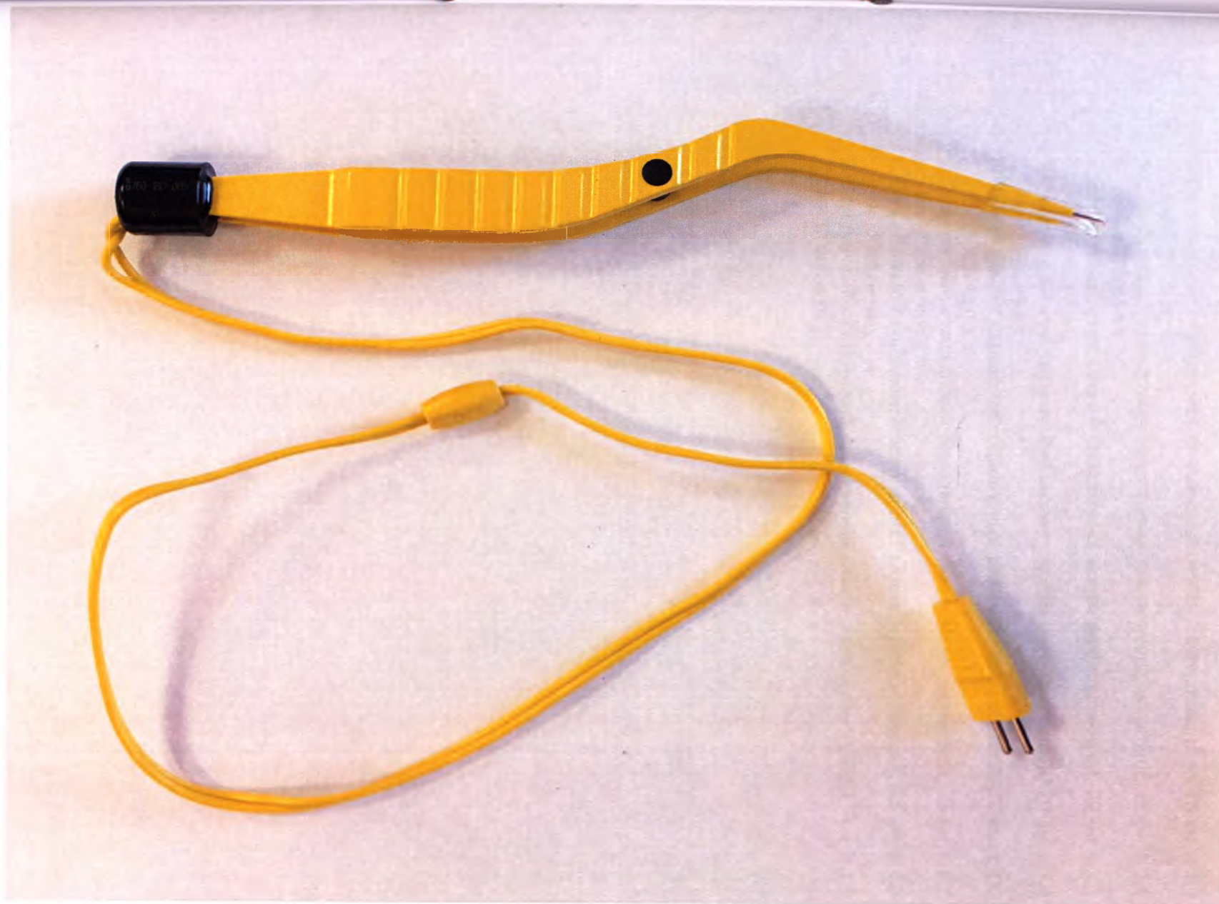
Рисунок 33 Одноразовый стандартный биполярный зажим неприлипающий, 18см x 0,5мм без упаковки
