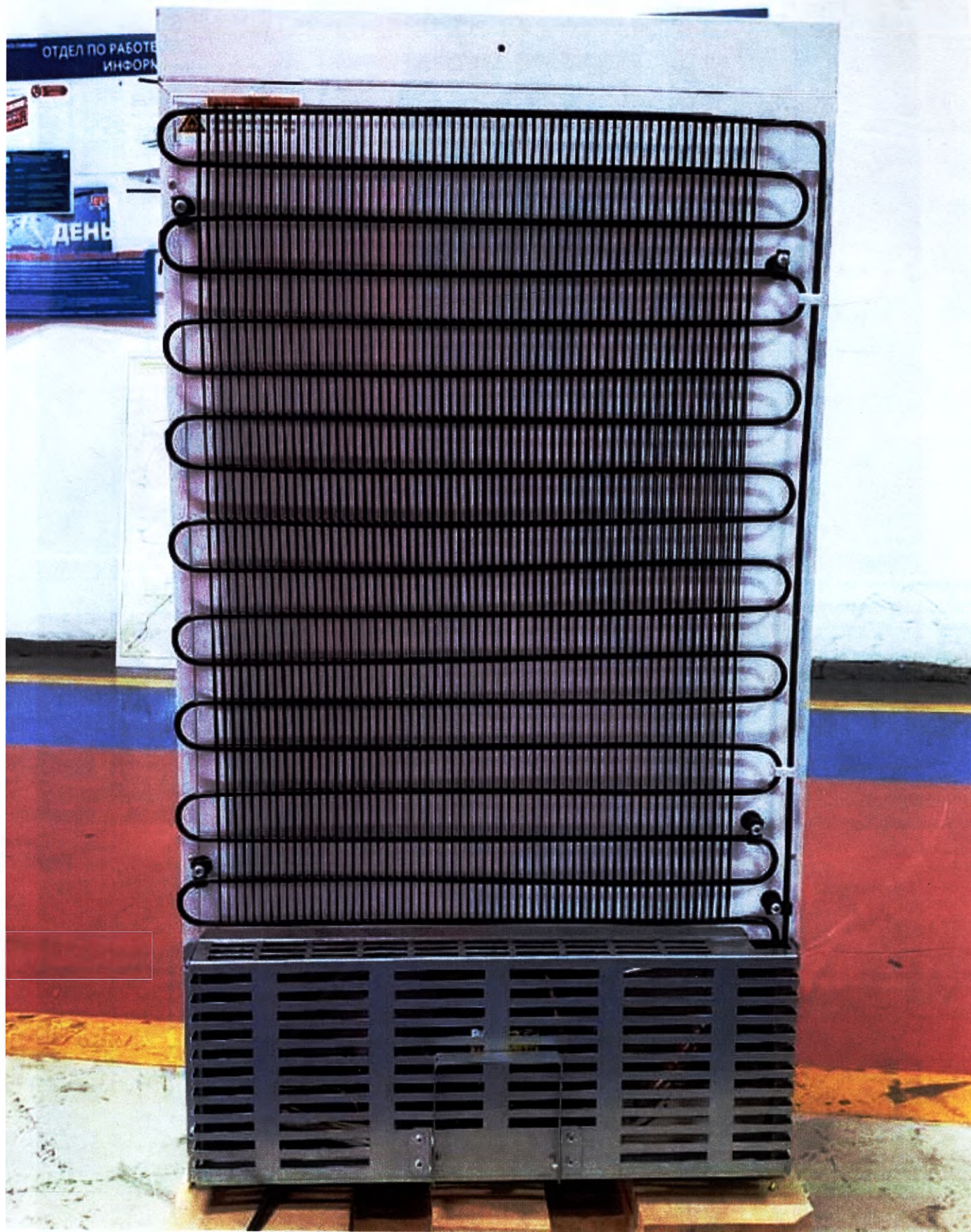
Холодильник фармацевтический «FRIGOGLASS» PH-150 [R600a] по ТУ 28.25.13-001-46204423-2021
