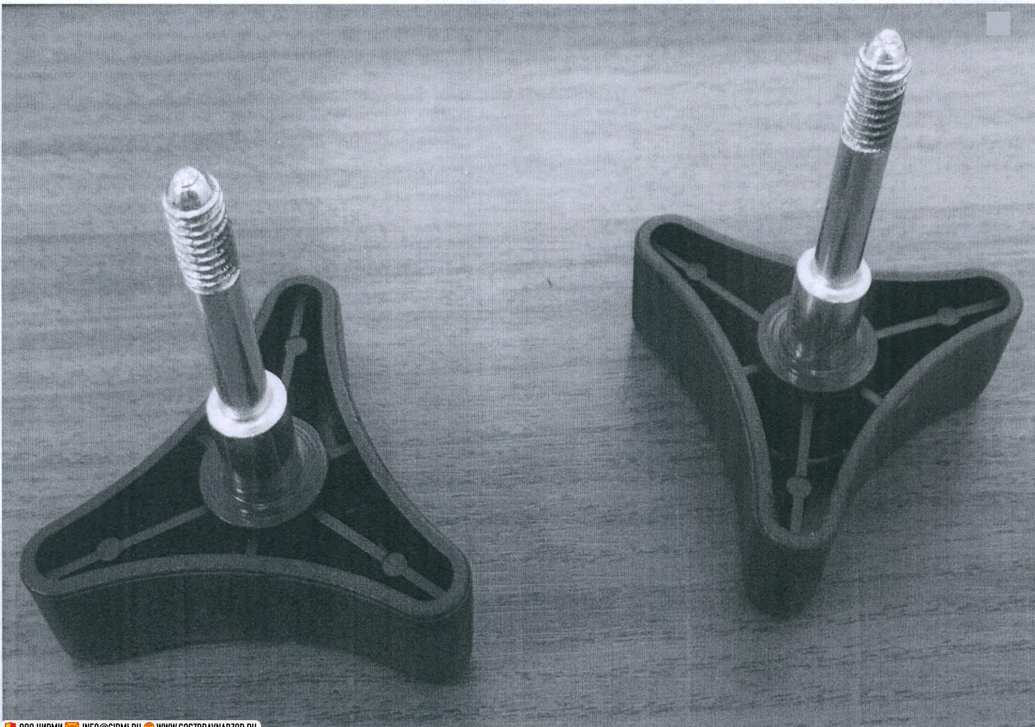
Рис. 57 – Винт-барашек (2 шт.)
