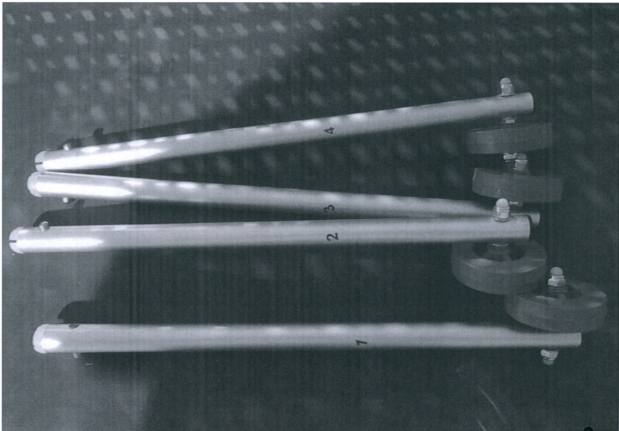
Рис. 65 – Ножка с колесиком (4 шт.)
