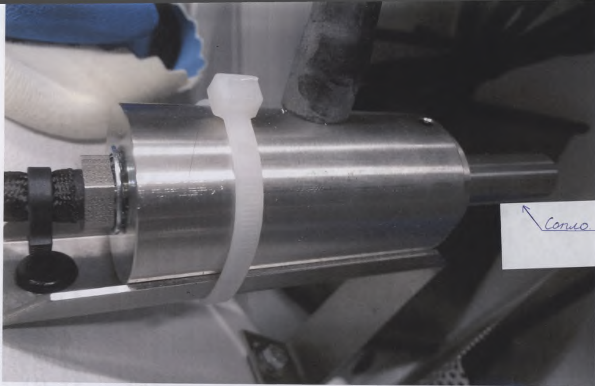
5. Принадлежности к Аппарату пескоструйному Vario jet для зуботехнических лабораторий: Сопло Blasting nozzle compl. f. 2960.
