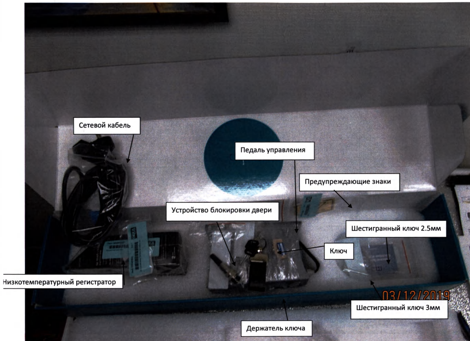
Система радиочастотная для коррекции контуров тела: аппарат радиочастотный для терапевтического использования Onda в составе с принадлежностями (принадлежности)
