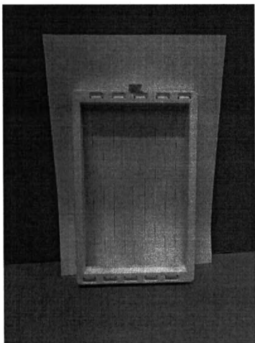
4. Коронирующая рамка
