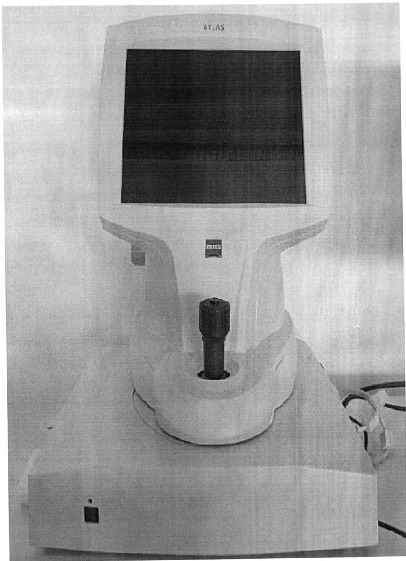
Корнеотопограф Atlas.
