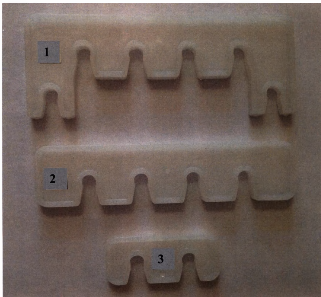
Держатель индуктора-кабеля №1, №2, №3
