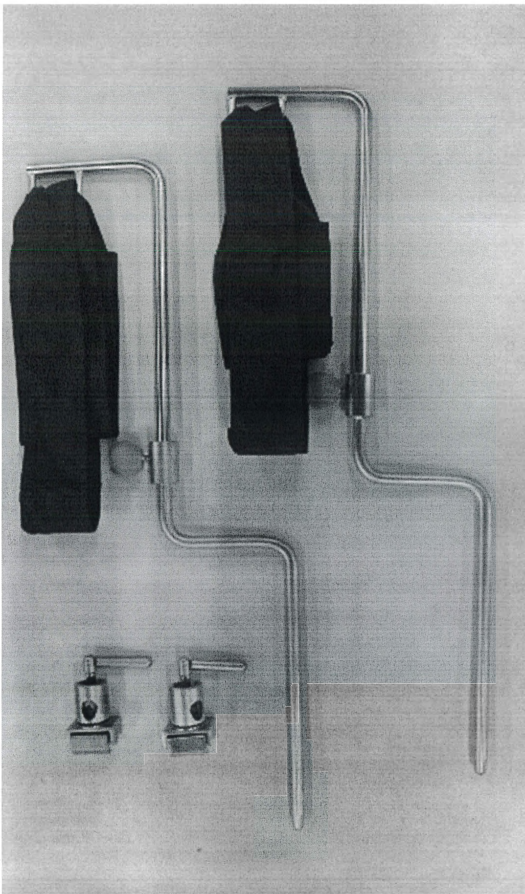
Опоры для ног с петлями
