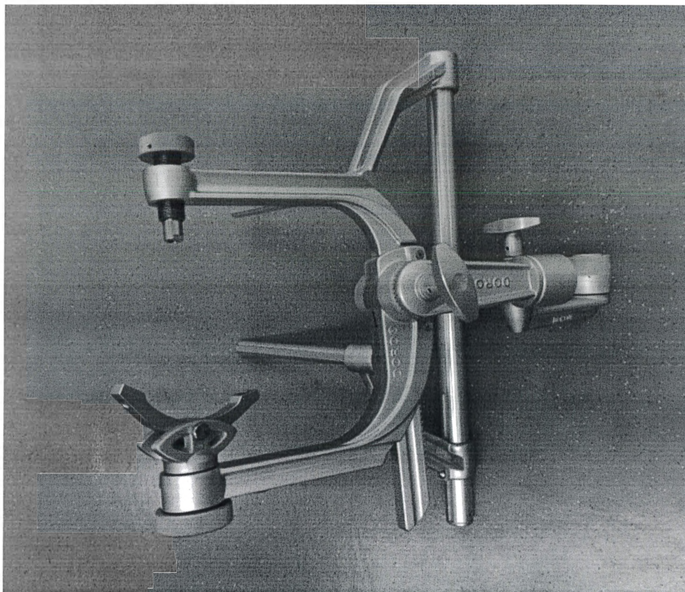
Фиксатор черепа нейрохирургический алюминиевый
