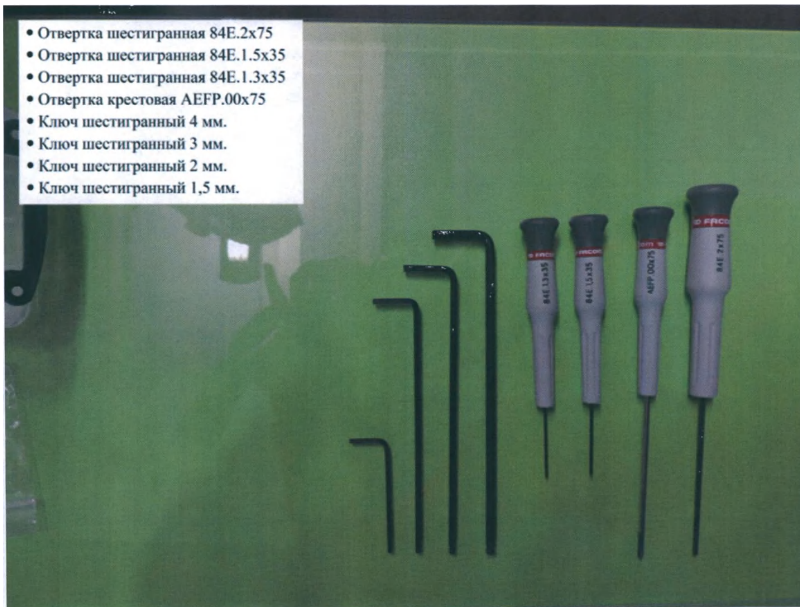
Фото 10. Набор для монтажа
