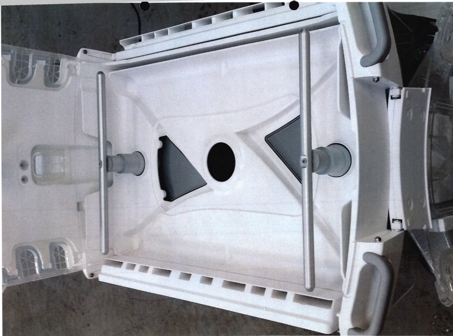
Блок измерения веса ребёнка (устанавливается во внутреннюю часть)
