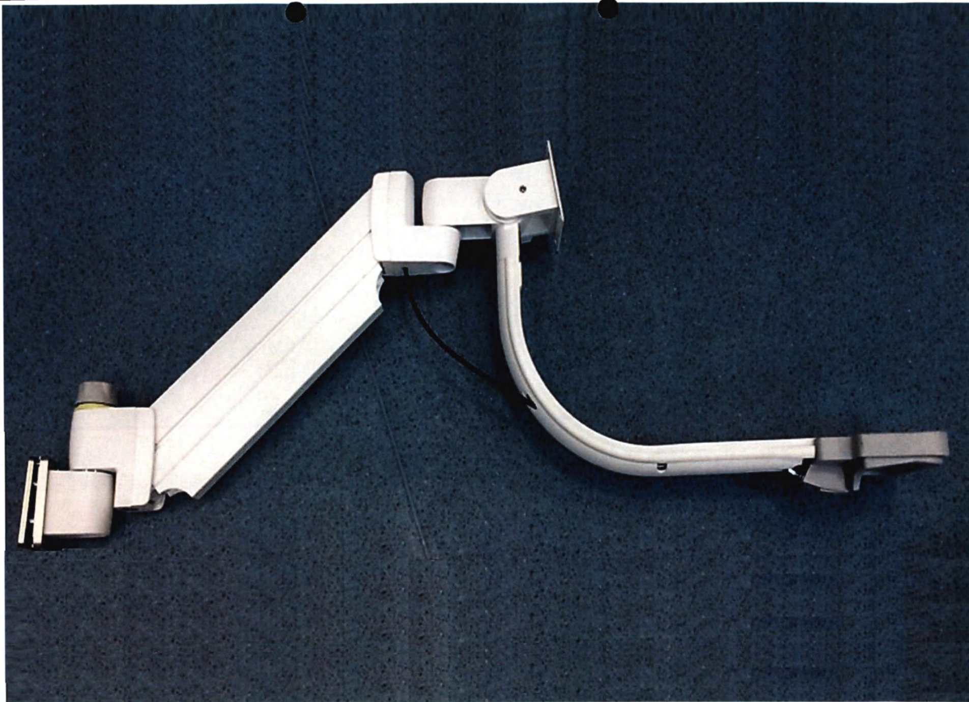
Кронштейн крепления дисплея с монтажным интерфейсом стандарта VESA с динамическим изменением положения и высоты
