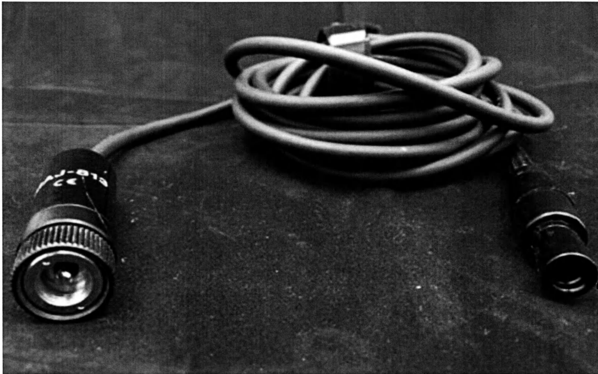
S-шнур МН-470, МАJ-813.
