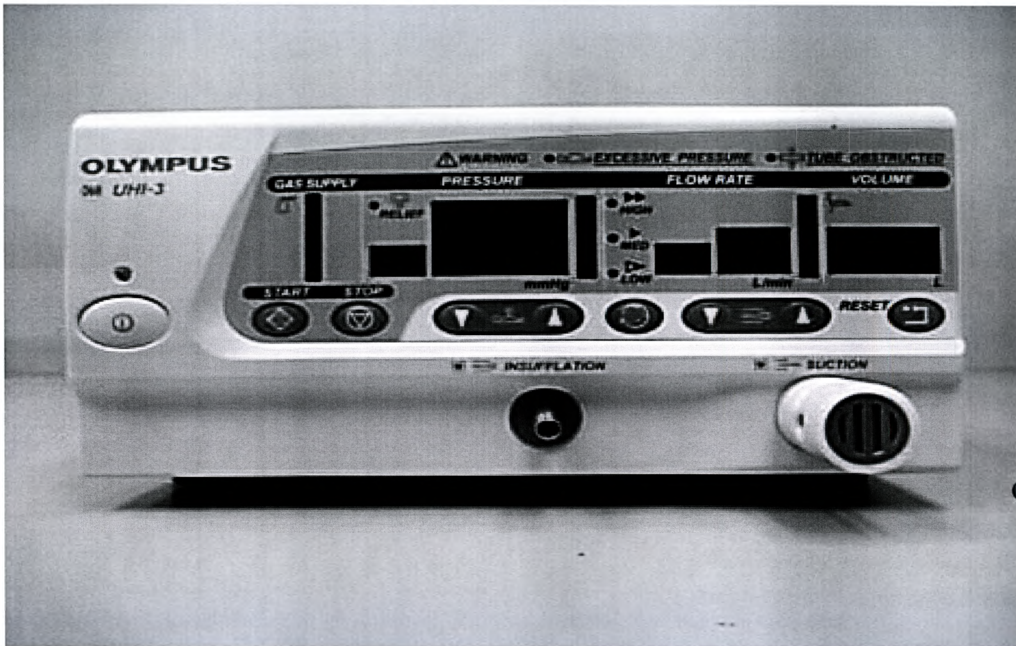
Инсуффлятор УНІ-3
