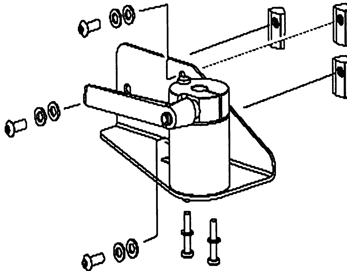
Опора держателя MAJ-1663.
